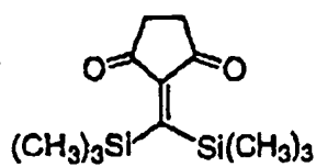
C-22
