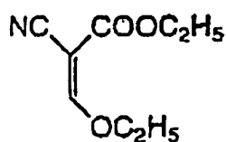
C-5
