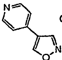
C-9
