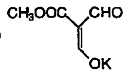
C-16
