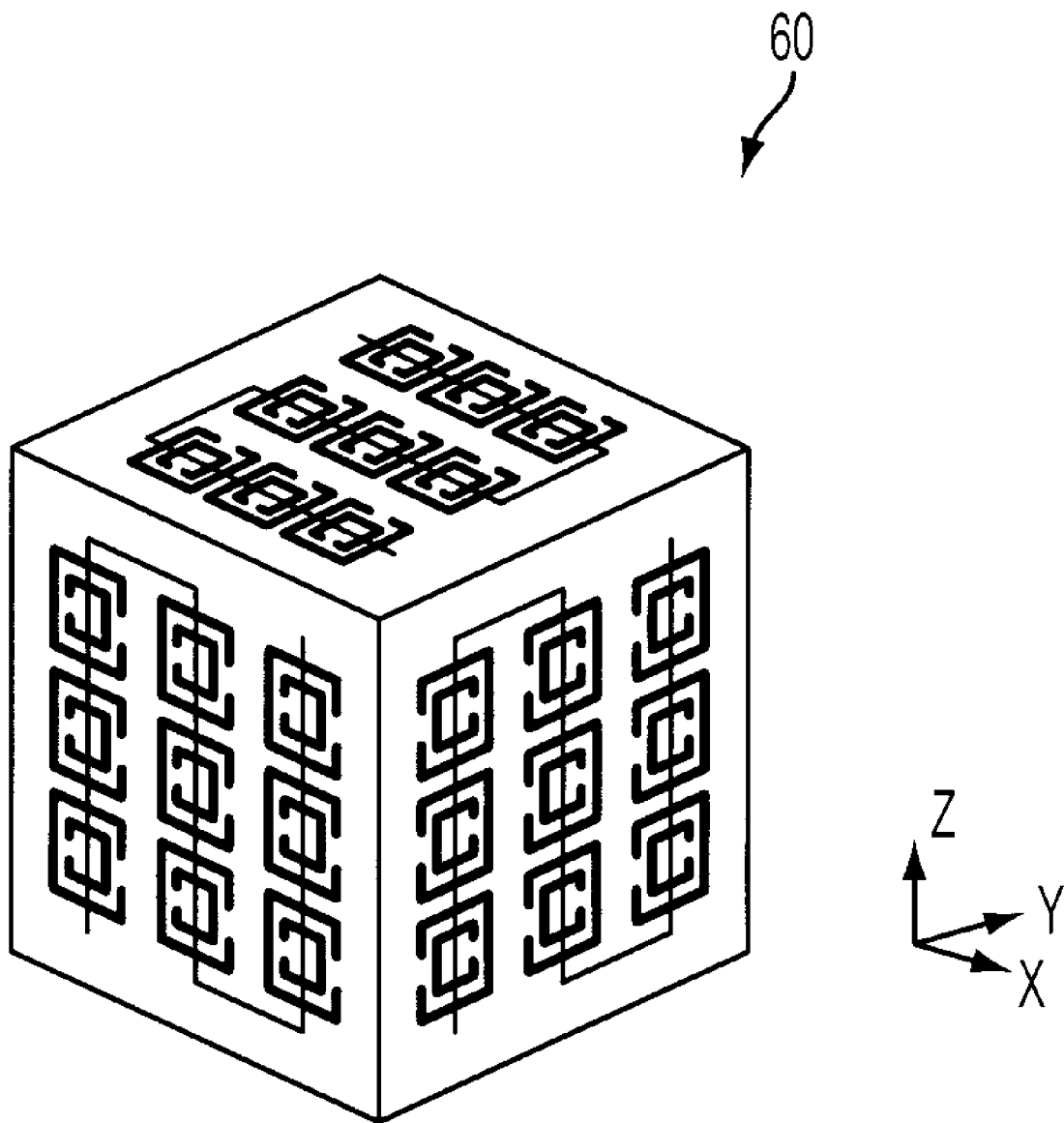
FIG. 6A
