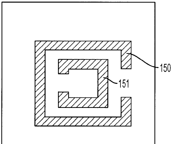
FIG. 4H
