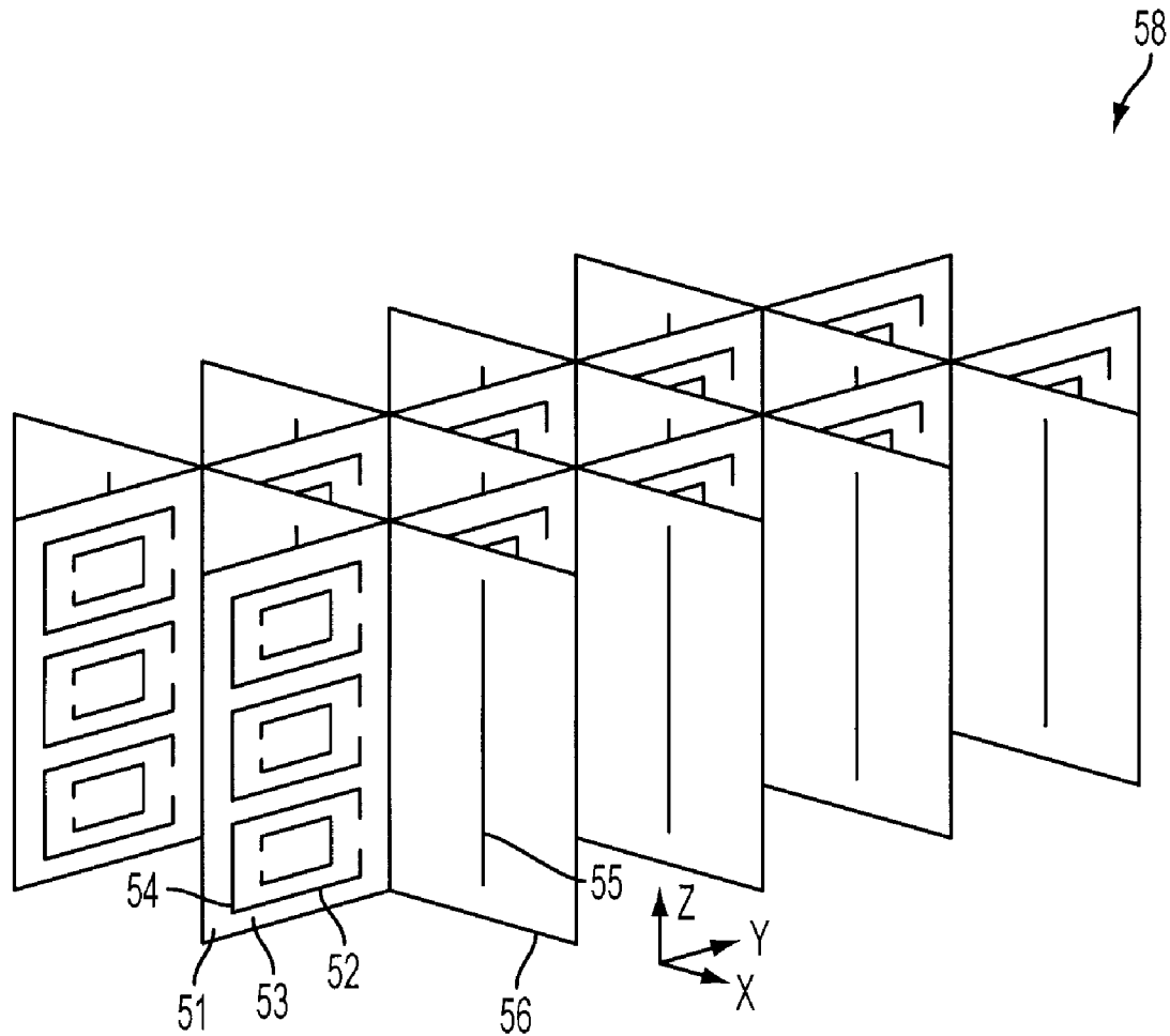
FIG. 5A
