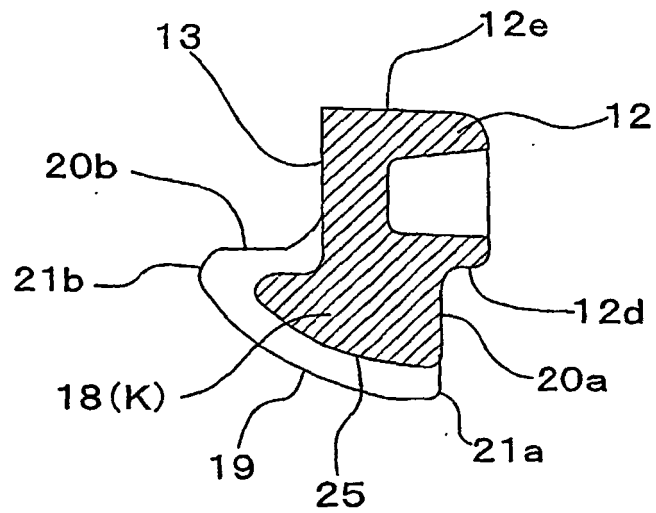
(a) C—C線切断矢視図
