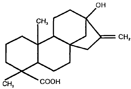
Steviol
