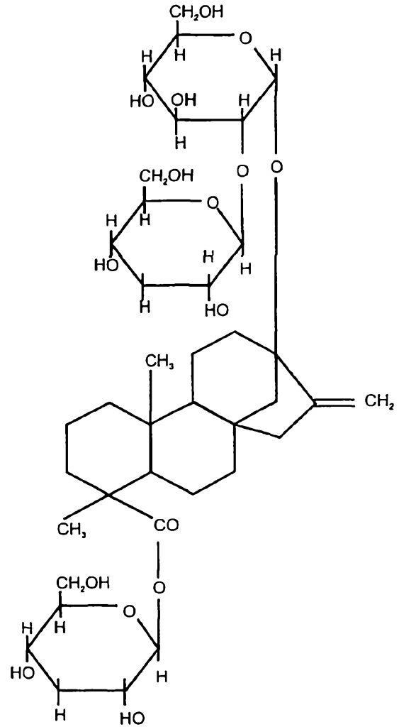
Stevioside
