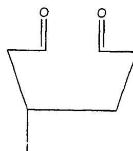
VIIc
