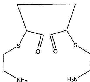
IXb
