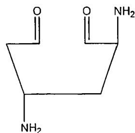
VIIIc
