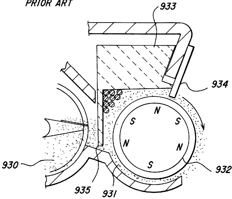
FIG. 25B PRIOR ART
