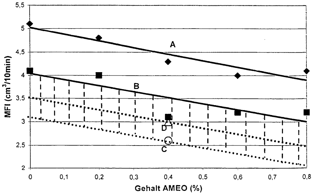
Bild 3) MFI-Werte als Funktion des Aminosilangehaltes.
