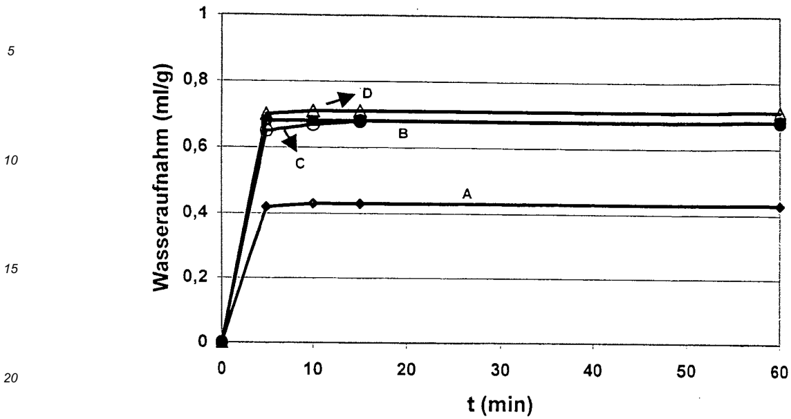
Bild 1) Wasseraufnahme nach Baumann für das erfindungsgemäße Produkt A und die kommerziell erhältlichen Produkte B, C und D.
