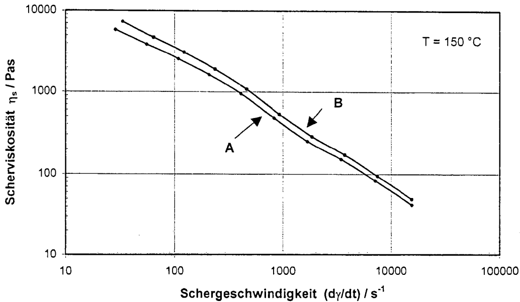
Bild 4) Scherviskosität der in Tabelle 8) aufgeführten Compounds.
