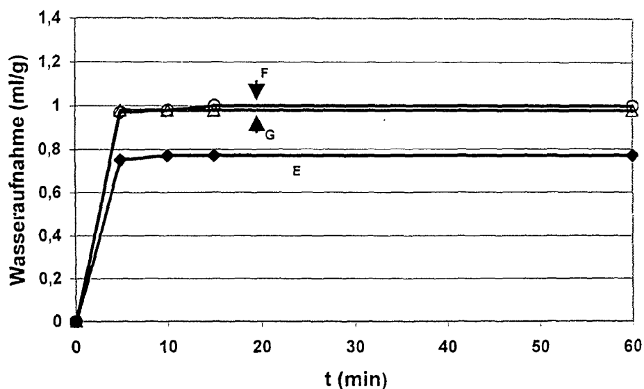
Bild 2) Wasseraufnahme nach Baumann für das erfindungsgemäße Produkt E und die Vergleichsprodukte F und G.
