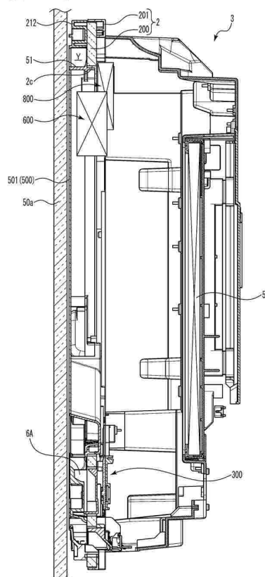
【图16-4】 A—A断面图
