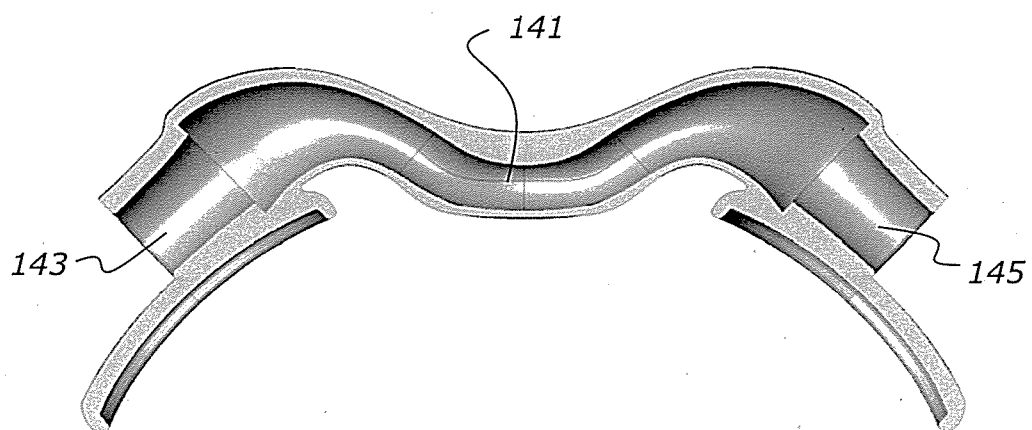
FIG. 11C
