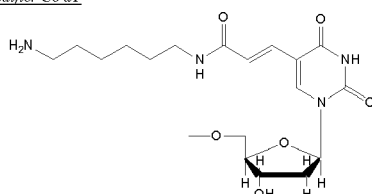
Amino modifier C6 dT
