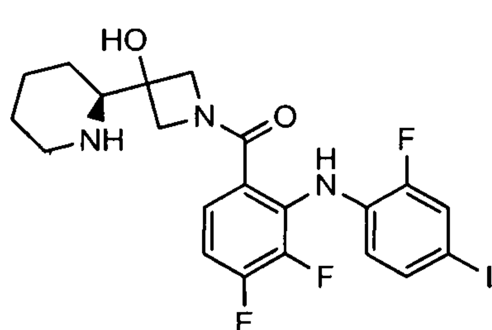
GDC-0973
