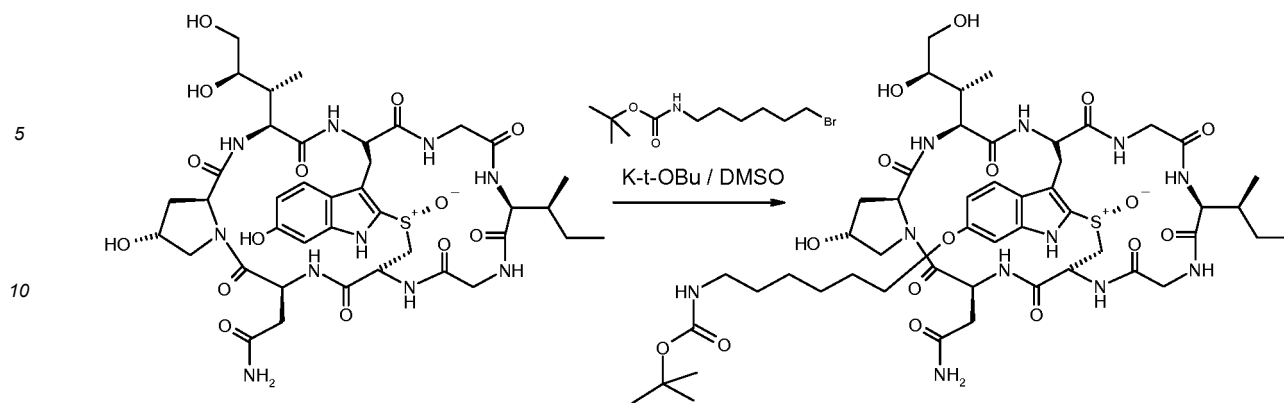
\alpha -amanitin
