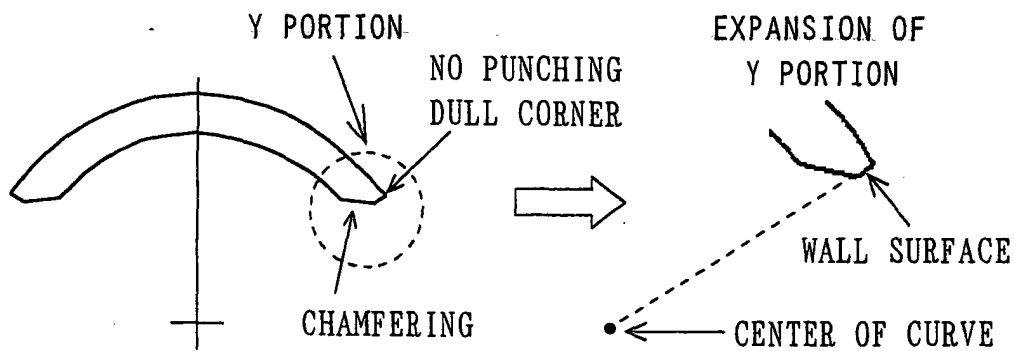
FIG. 16 (D) SHAPE OF COMMUTATOR ELEMENT
