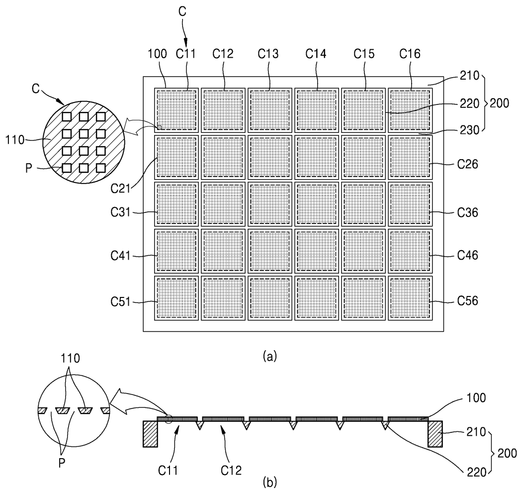
도면4
