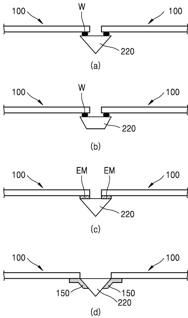
도면8
