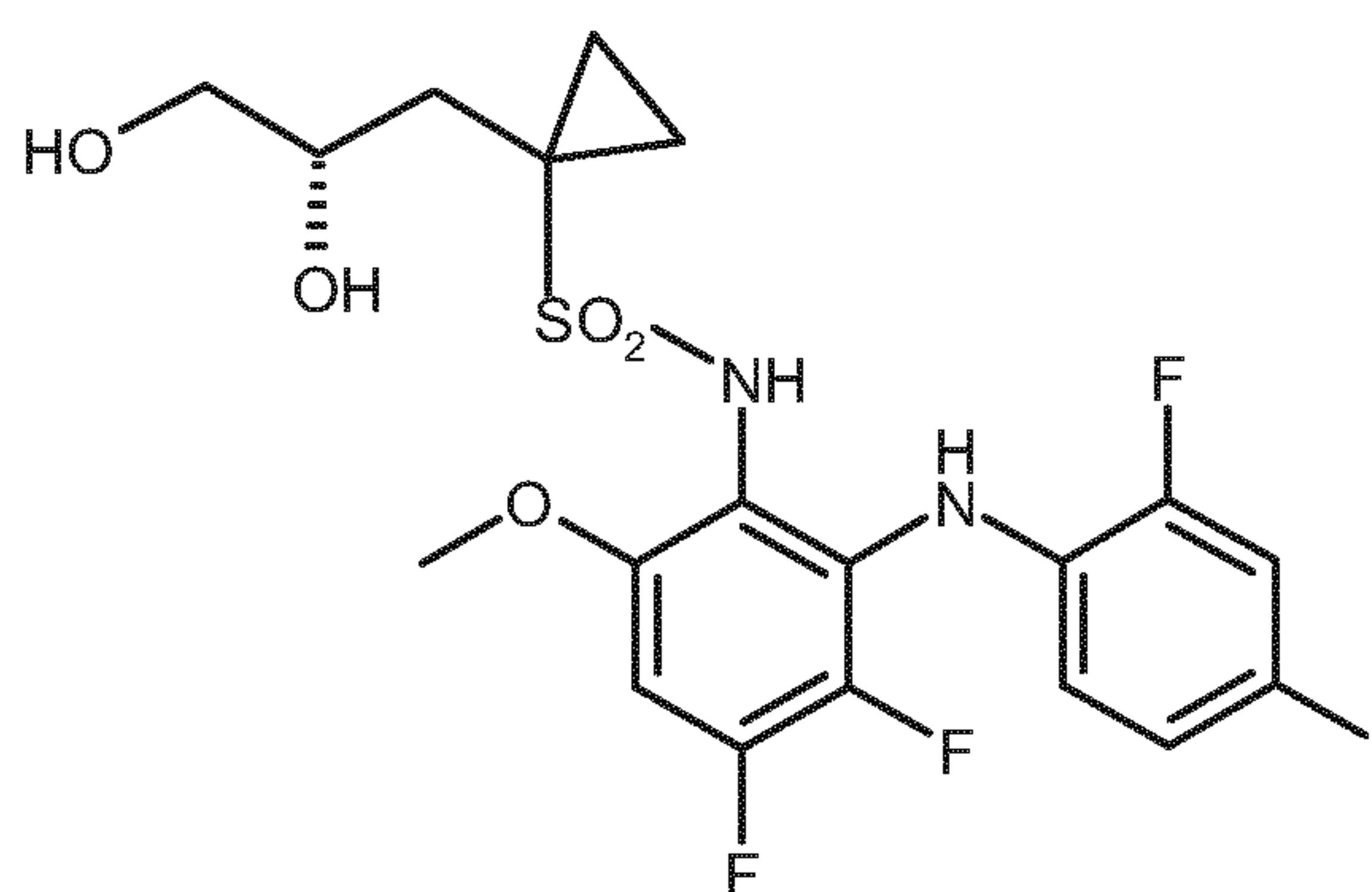
(S)-14 ;
