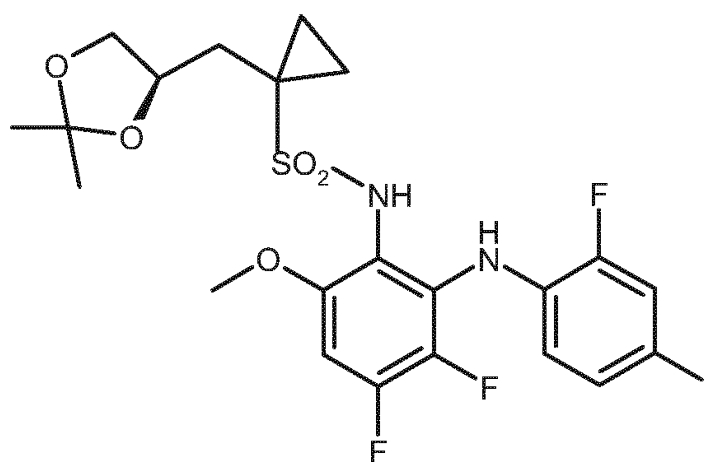
((R)-13)
