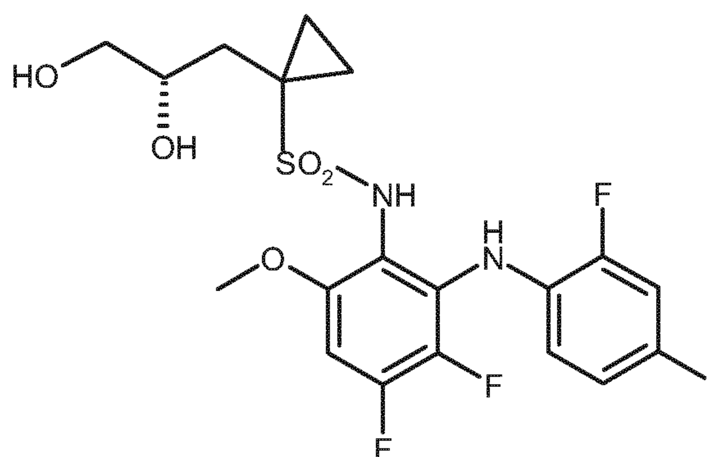
(S)-14 ;
