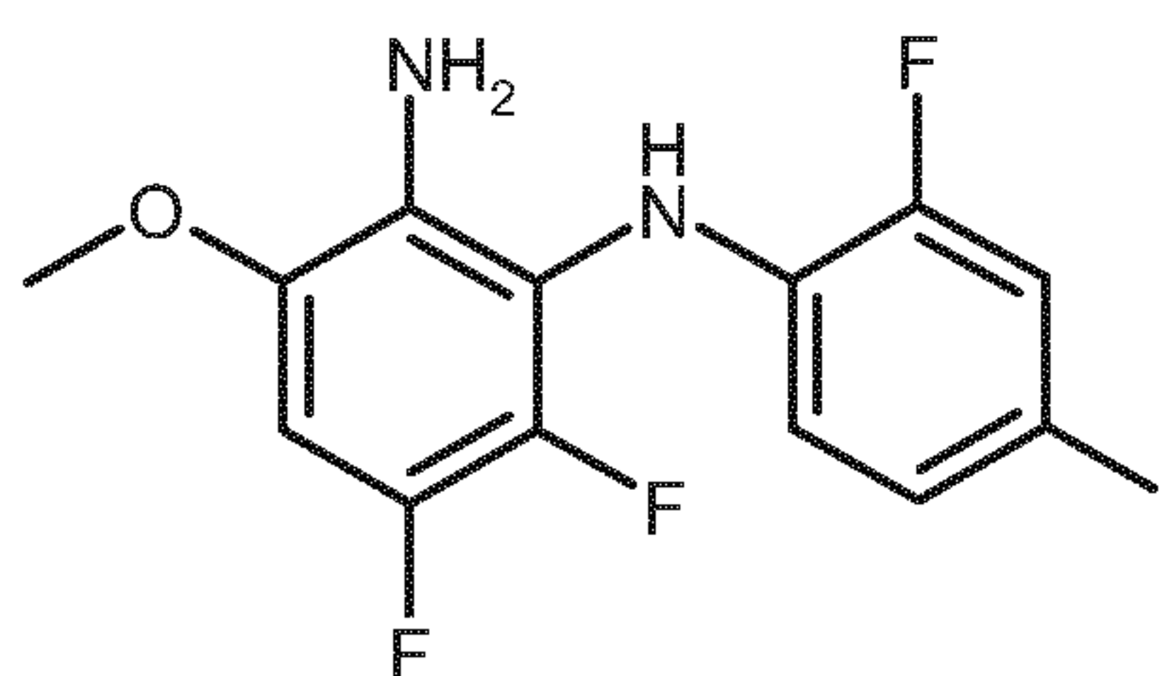
(12)
