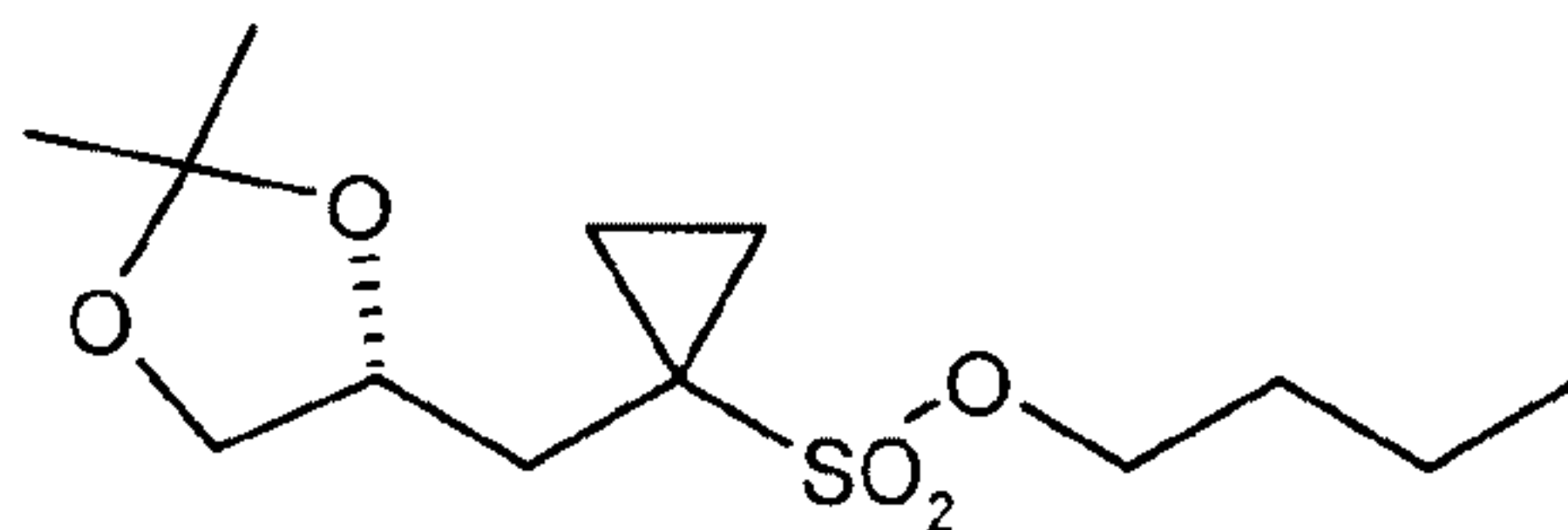
(R)-6 ;
