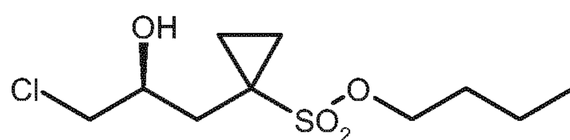
(S)-3 ;
