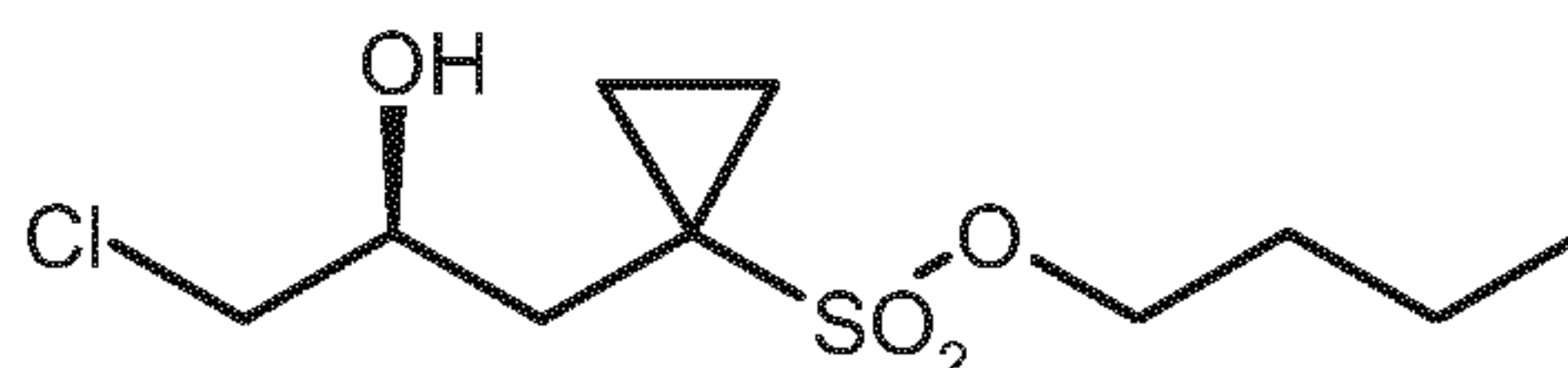
(S)-3 ;
