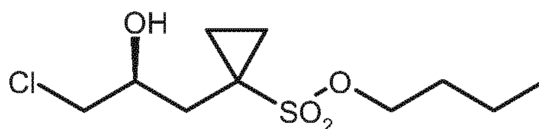
(S)-3 ;
