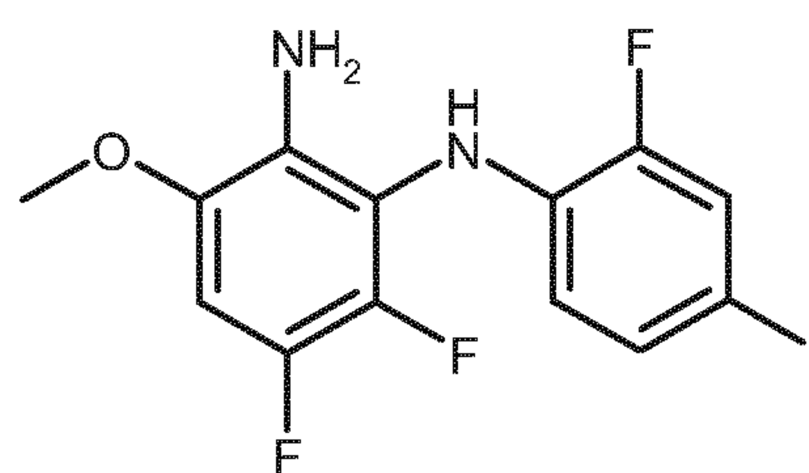
(12)
