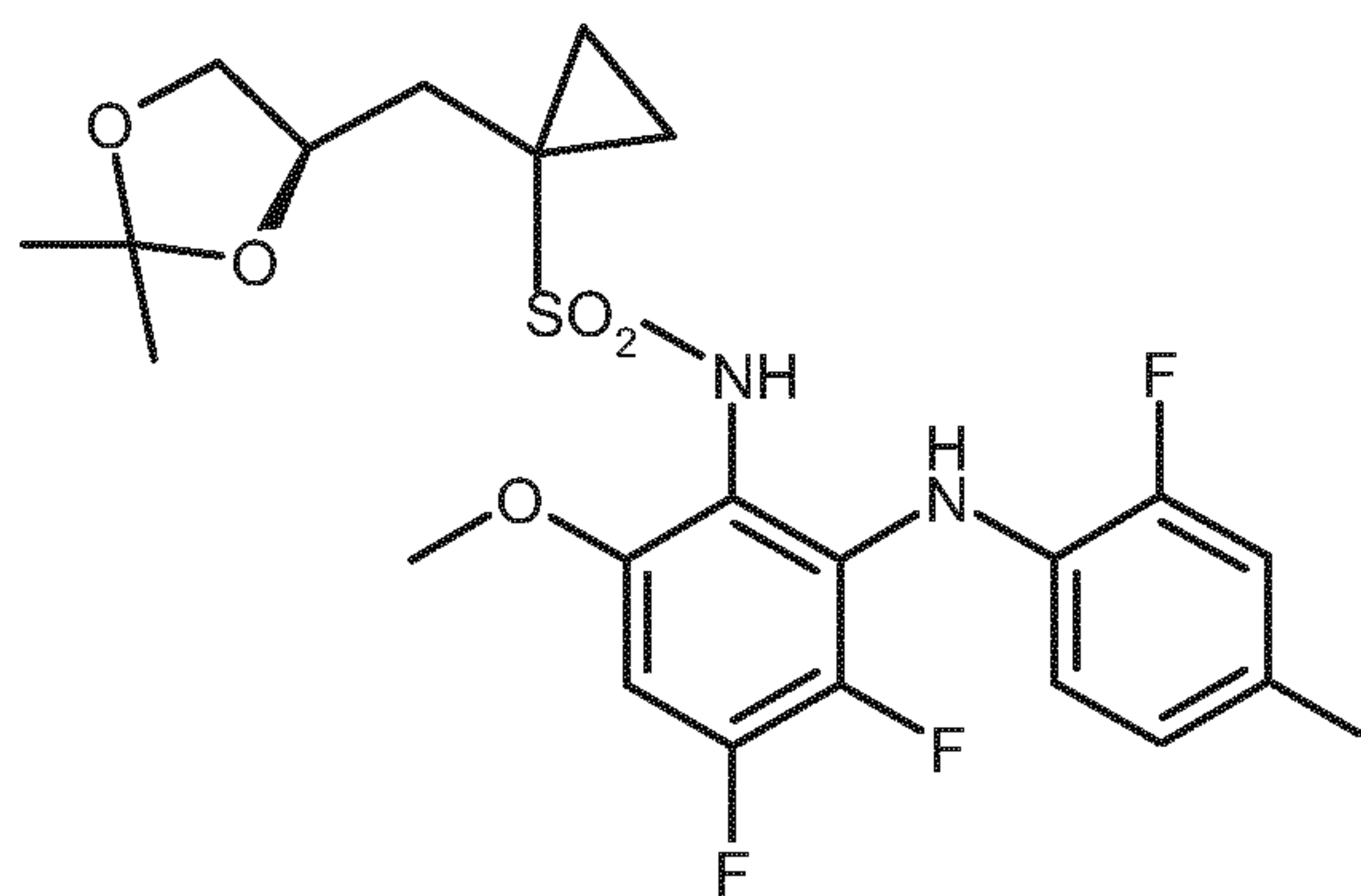
((R)-13)
