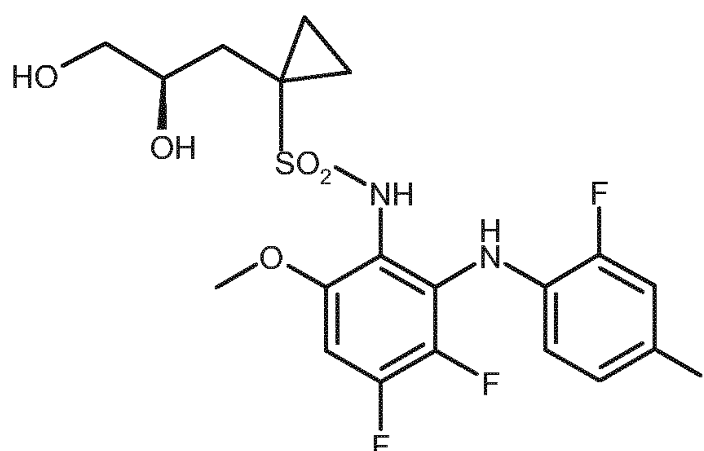
(R)-14 ;
