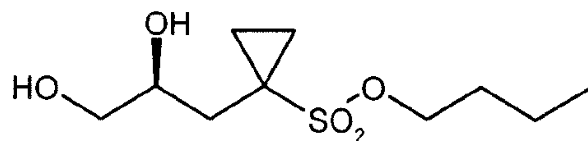
(S)-5 ;
