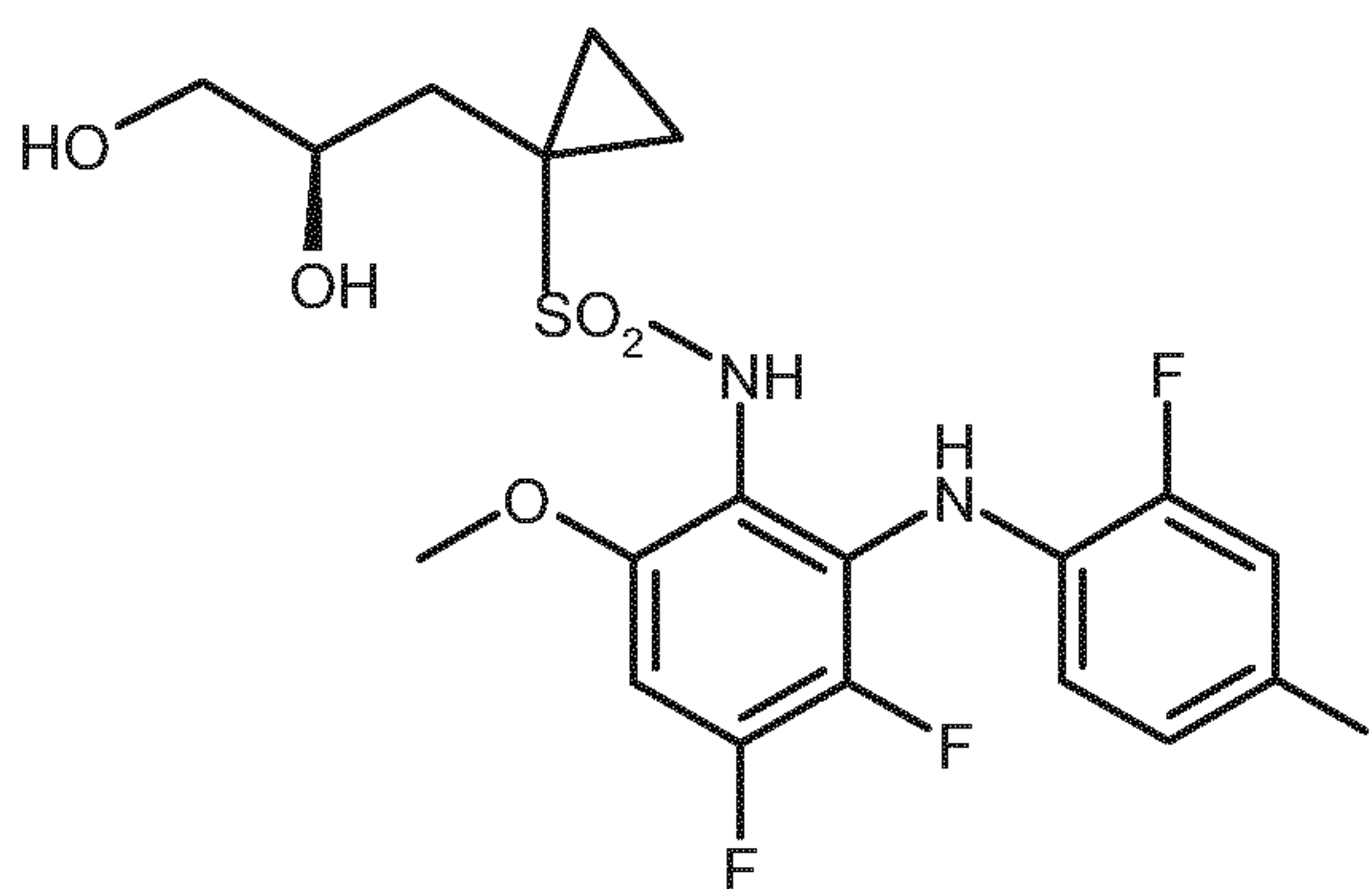
(R)-14 ;
