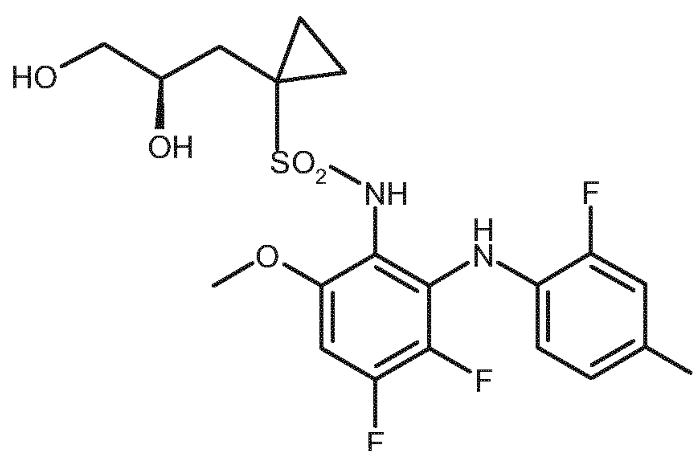
(R)-14 ;
