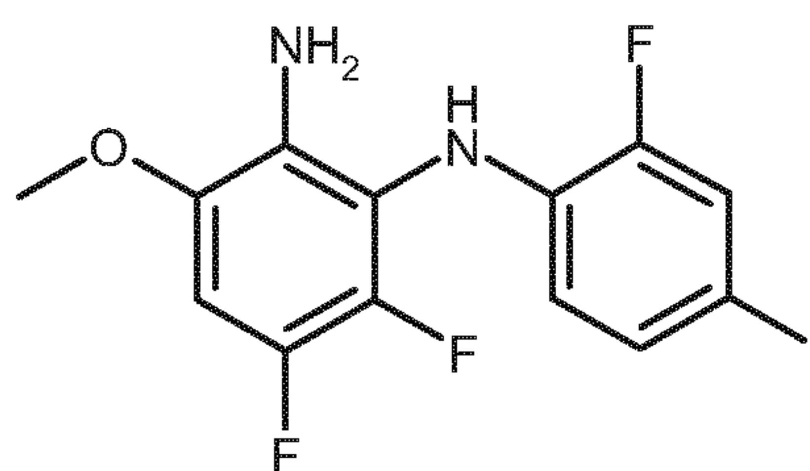
(12)
