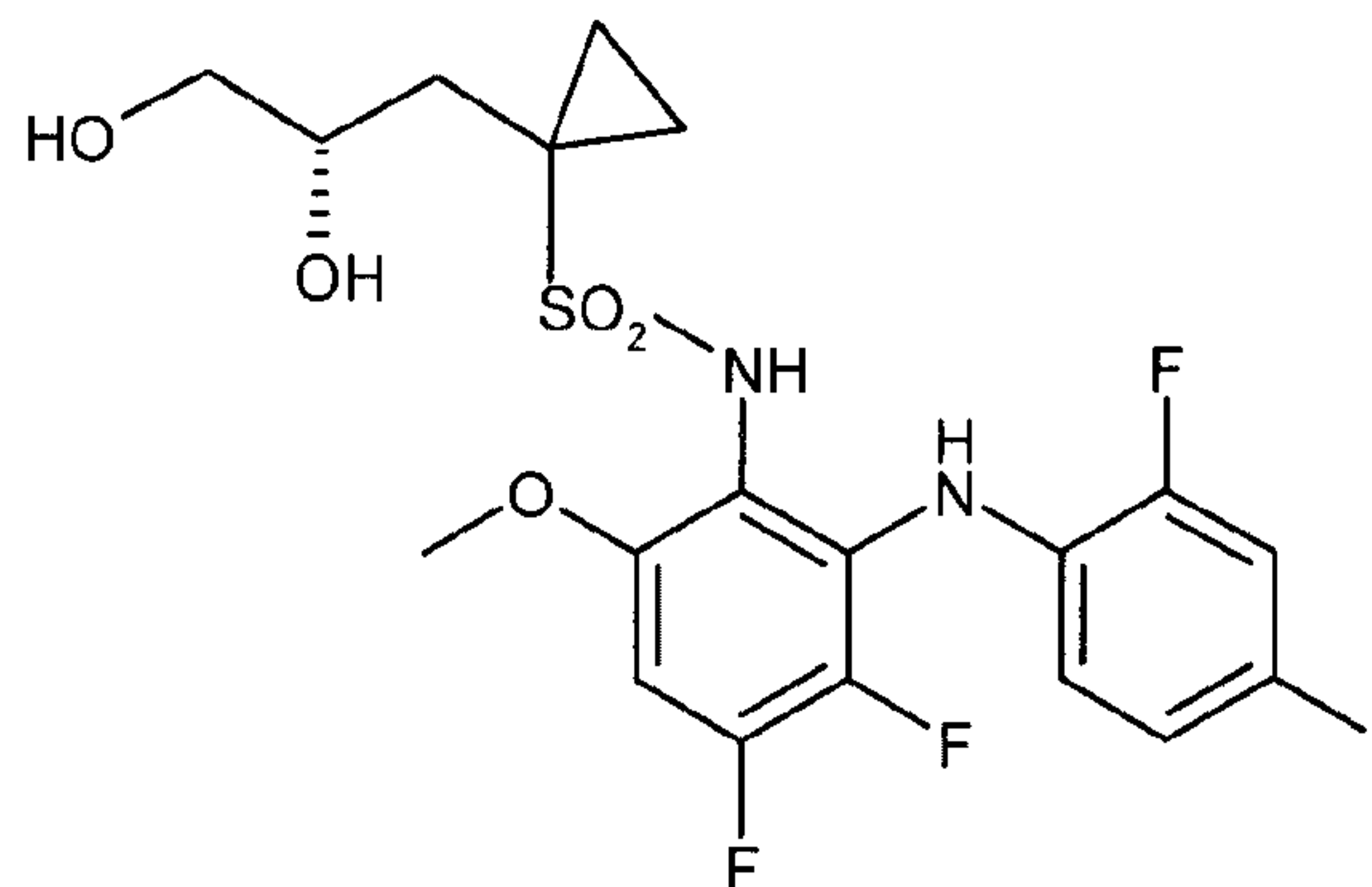
(S)-14 ;
