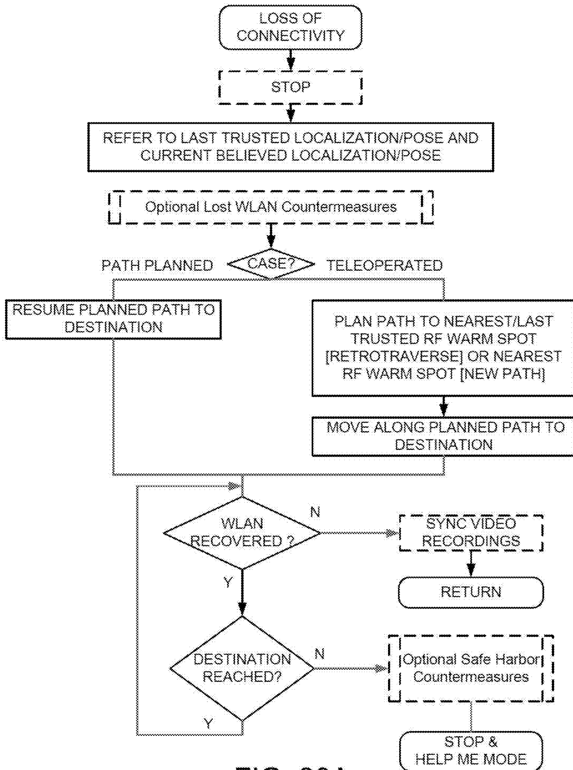
FIG. 20A
