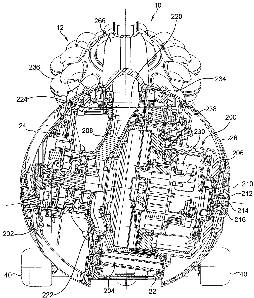
FIG. 23
