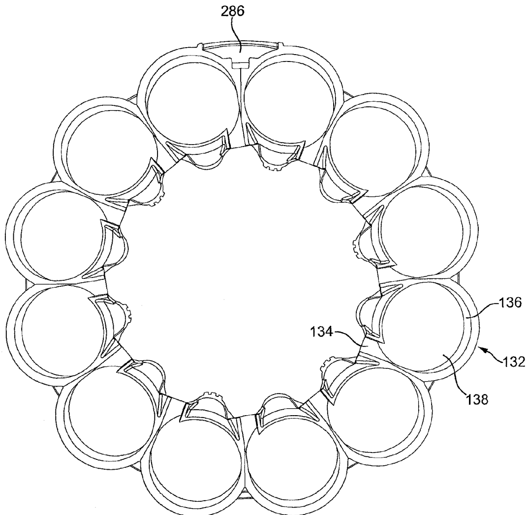
FIG. 14(a)
