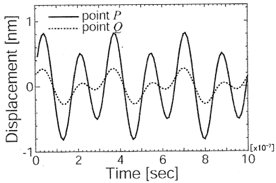
P点, Q点の変位図 (x軸方向)
