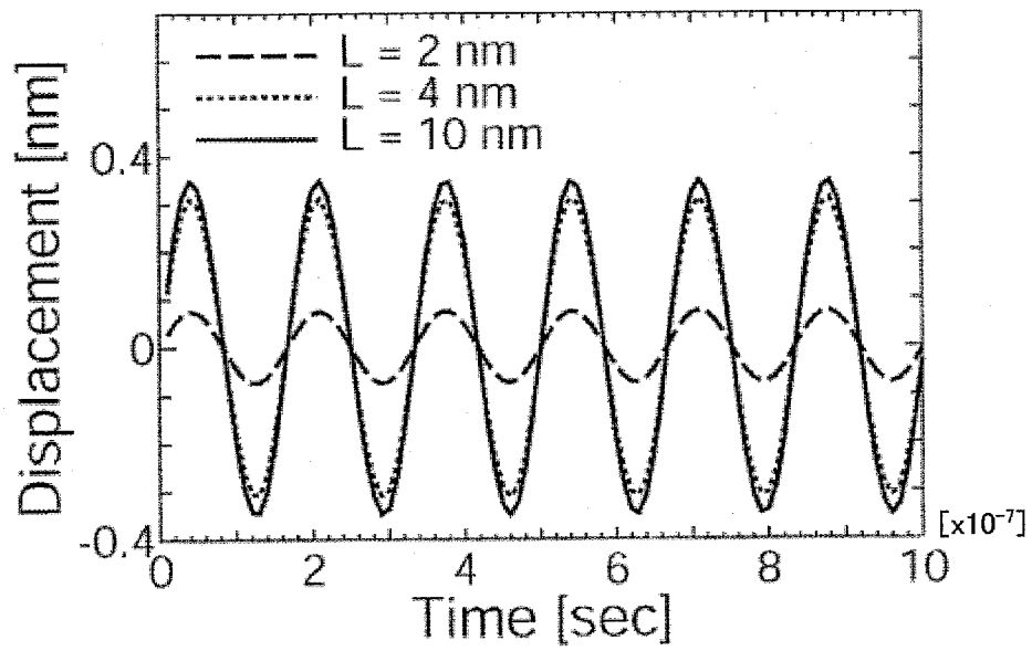
P点の変位図（ x 軸方向）
