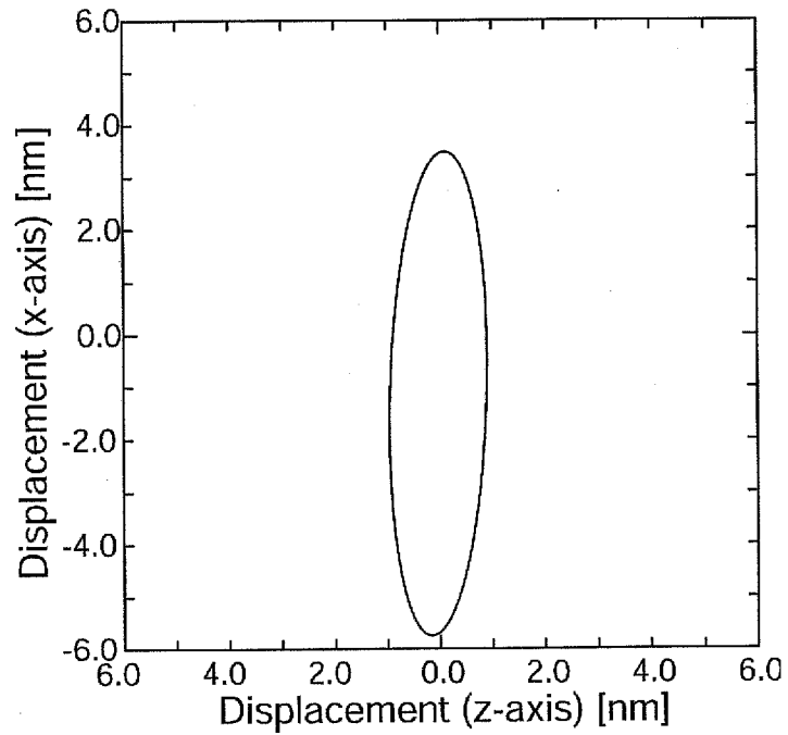
(b) 軌跡
