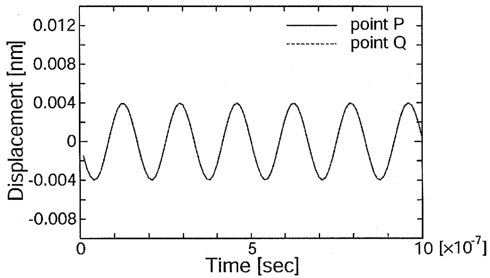
P点, Q点の変位図 (z軸方向)
