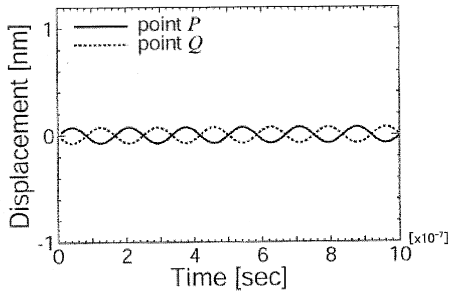
P点, Q点の変位図 ( x 軸方向)
