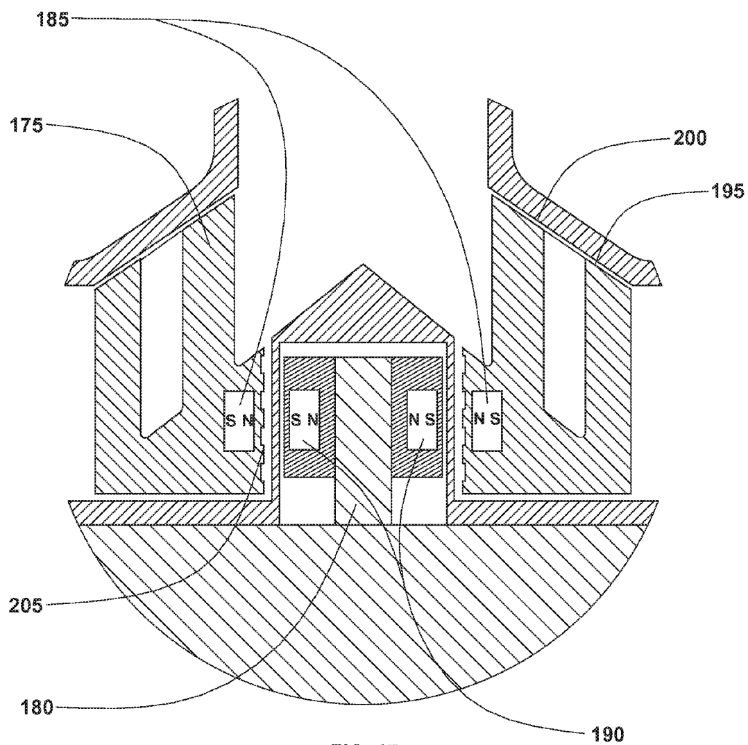
FIG. 17 (DETAIL E)
