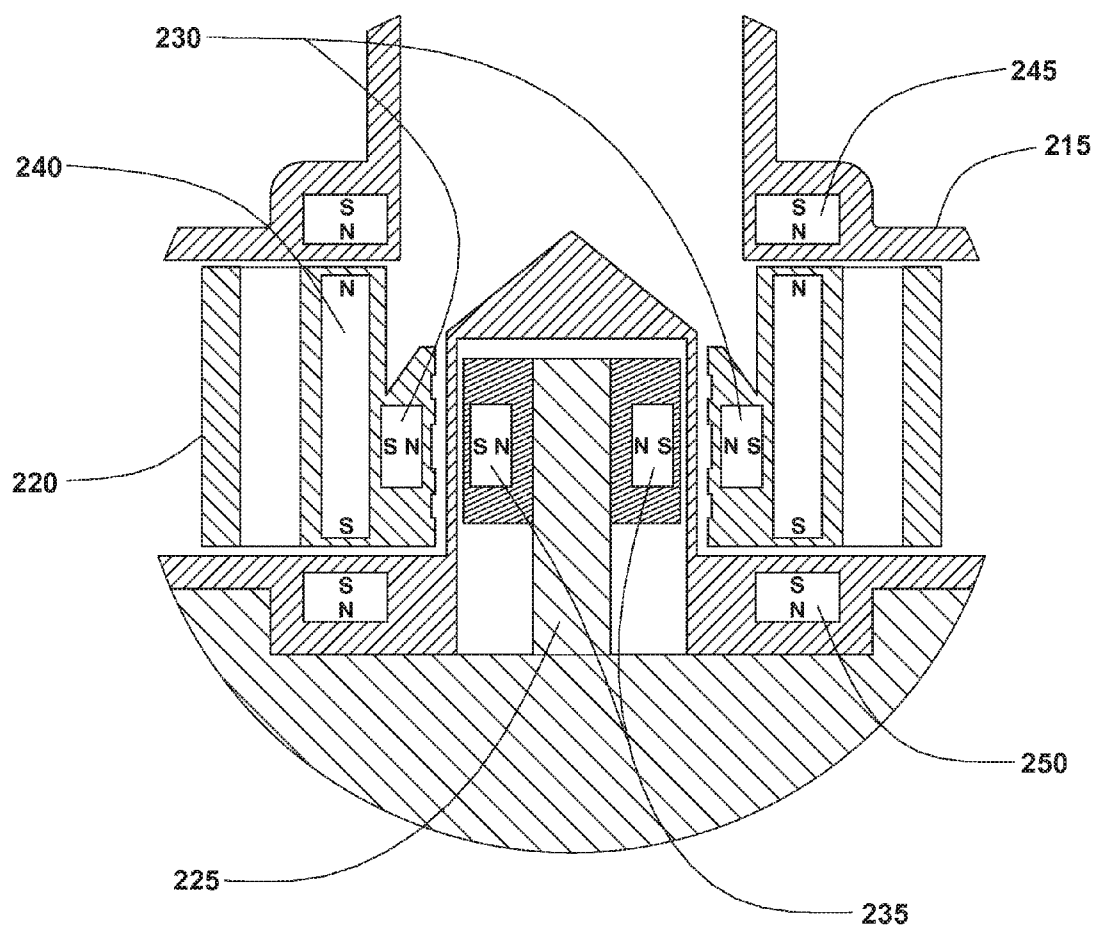
FIG. 20 (DETAIL H)
