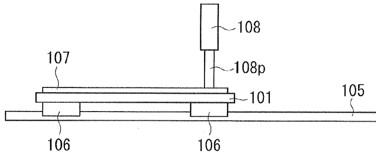
F I G . 7 B
