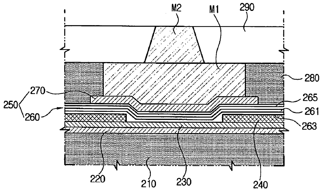
FIG. 4H
