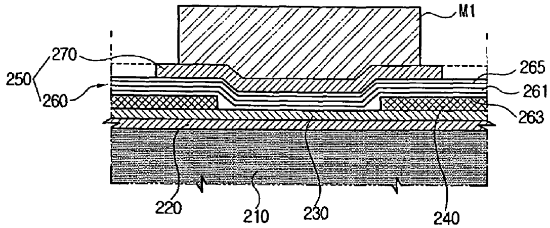
FIG. 4F
