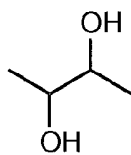
2,3-Butanediol
