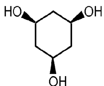
cis-1,3,5-Cyclohexanetriol
