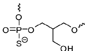
1,3,4- Isobutanetriol
