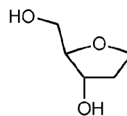
1,2-Dideoxyribose
