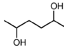
2,5-Hexanediol
