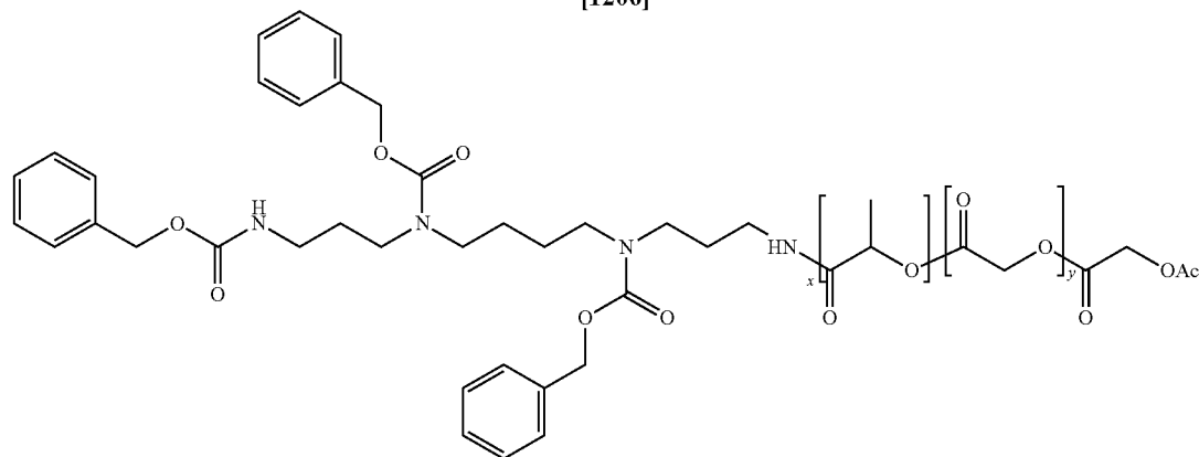
N1-PLGA-N5,N10,N14-tri-Cbz-spermine
