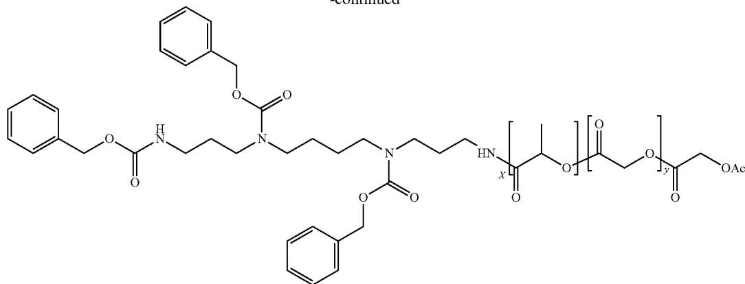
N1-PLGA-N5,N10,N14-tri-Cbz-spermine
