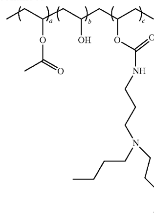
PVA-DBA
