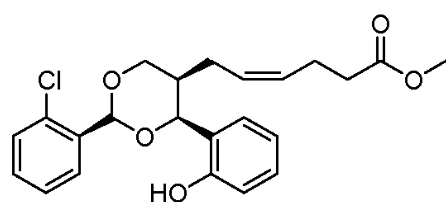
Prodrug 2
