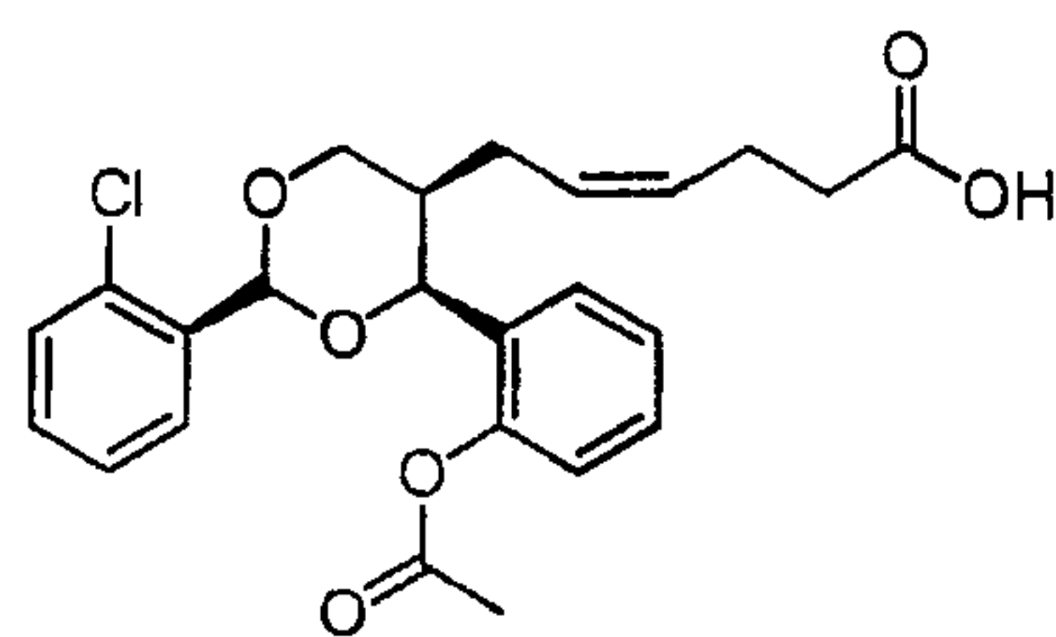
Prodrug 1
