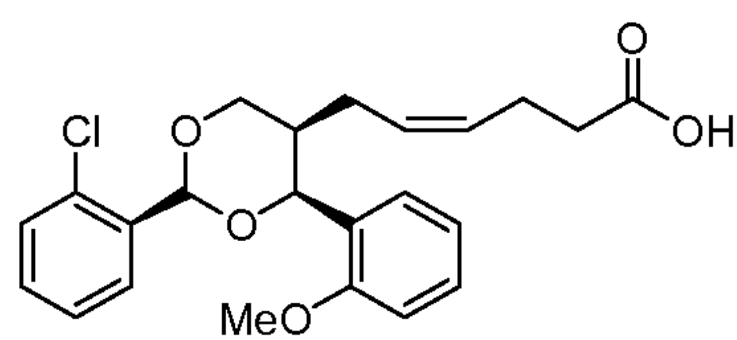
Prodrug 3
