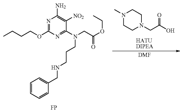
Scheme 107:
