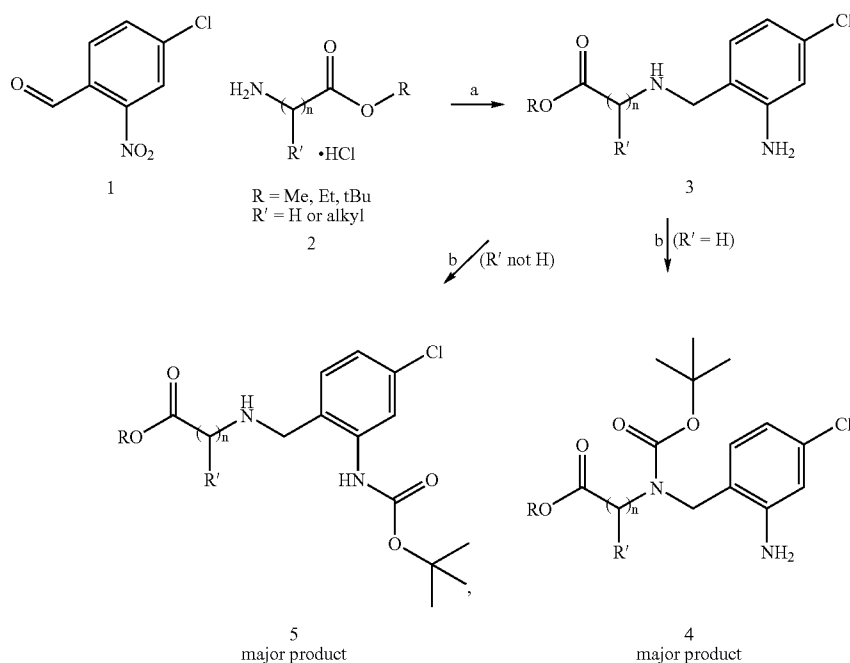
Scheme 5a.
