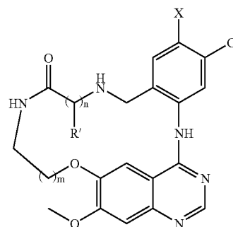
15b
