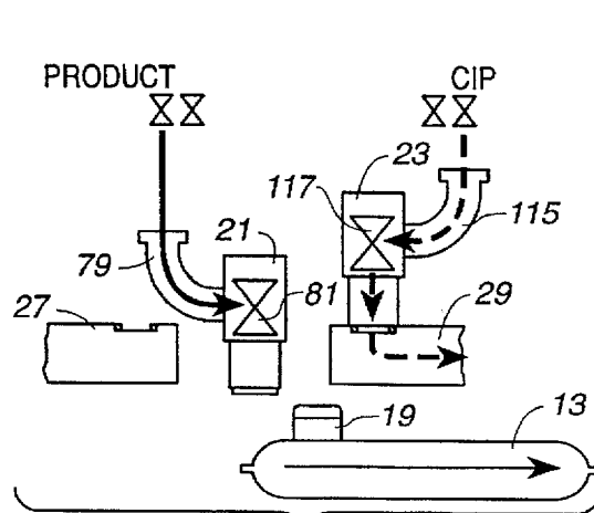
FIG. 3E
