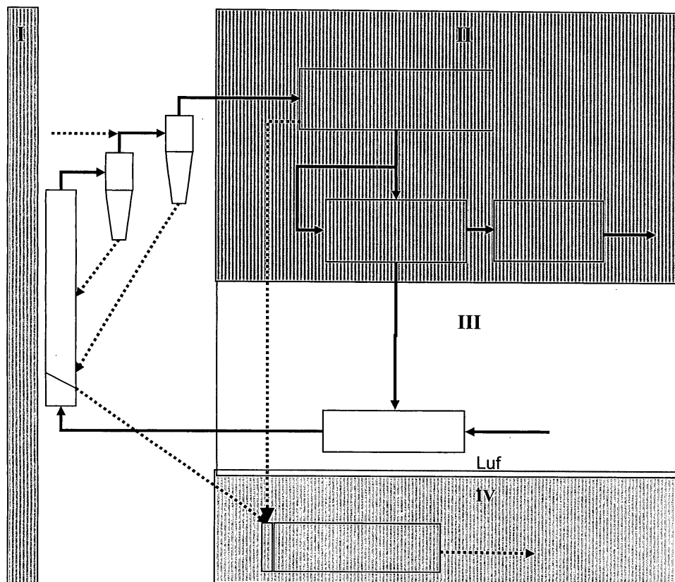
Fig. 1: Prinzipskizze der zirkulierenden Wirbelschichtanlage
