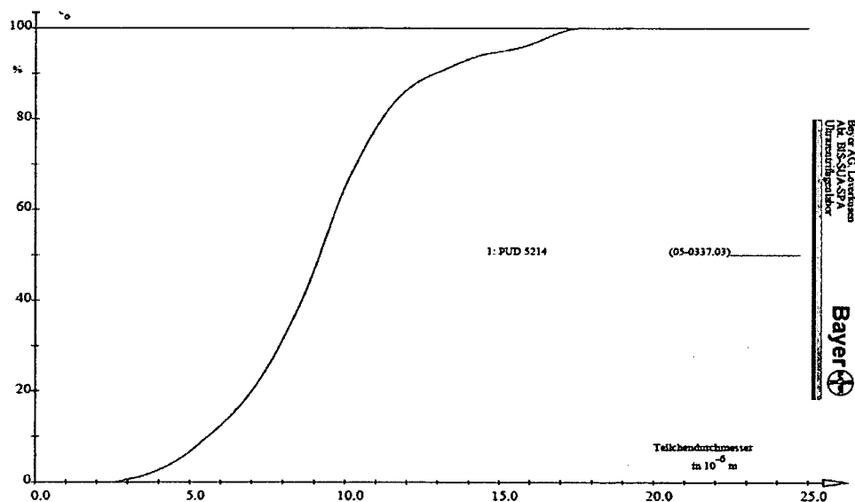
Teilchengrößenverteilung der PHMB Suspension aus Beispiel 2 mittels Ultrazentrifuge
