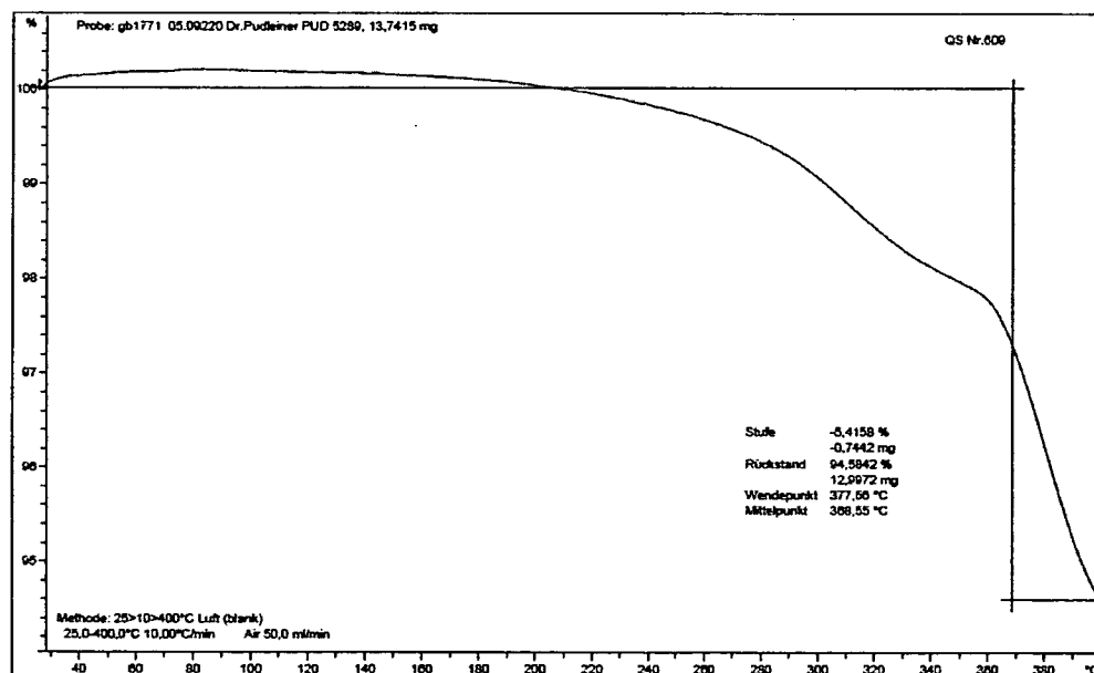
TGA-Kurve der Suspension aus Beispiel 1
