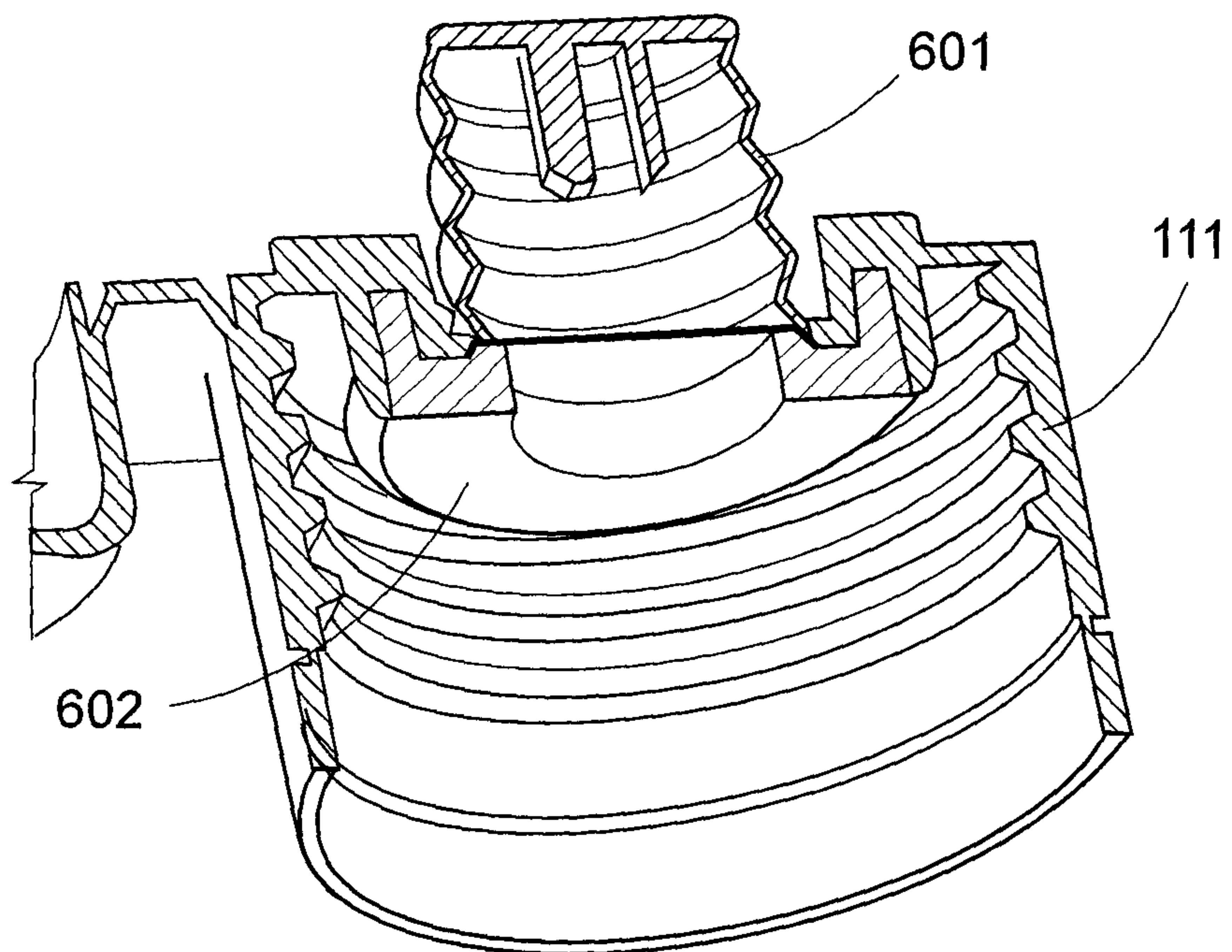
FIG. 6B
