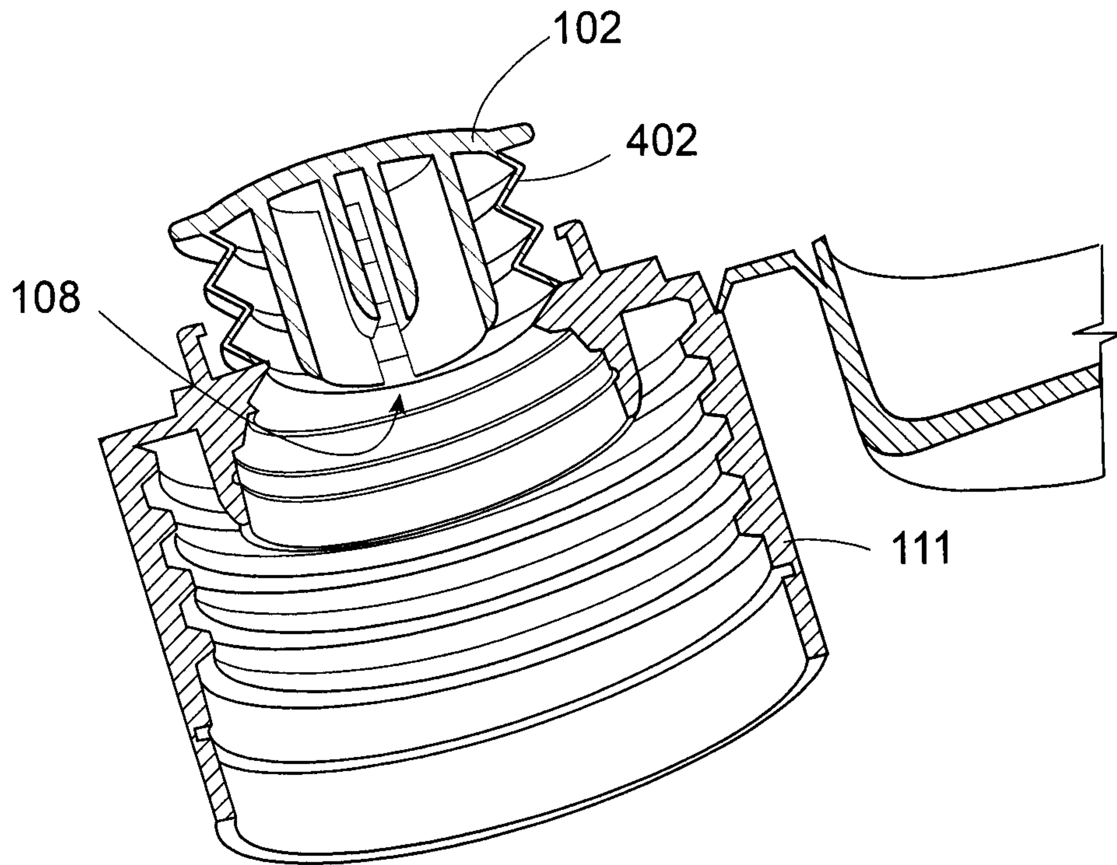
FIG. 5A
