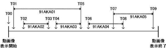
(A1) テキスト表示プロセステーブル91AKT01の場合
