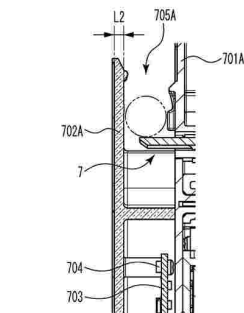
(C) 可変入賞球ユニット700
