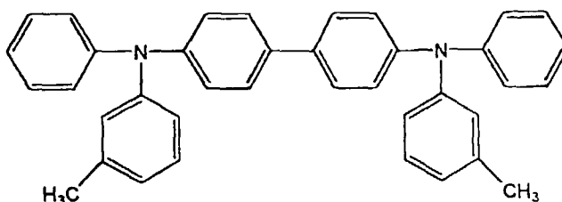
TPD
