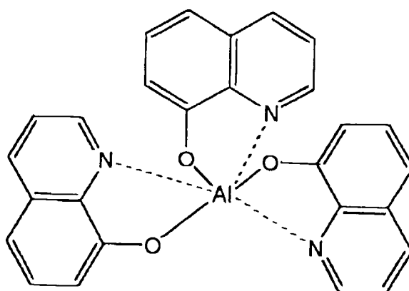
Alq3
