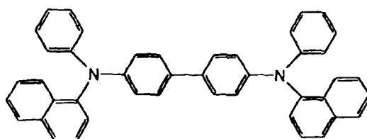
\alpha -NPD
