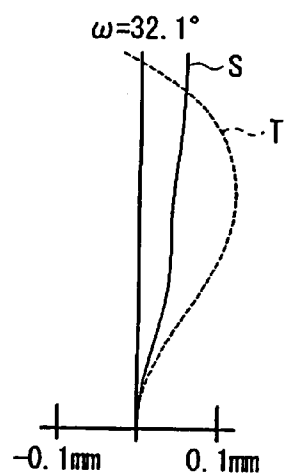
Astigmatism Fig. 3B
