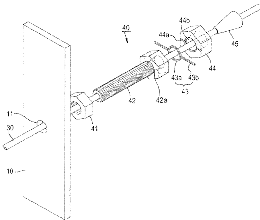
FIG. 1E (RELATED ART)
