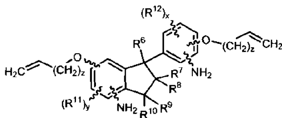
Struktur (I)
