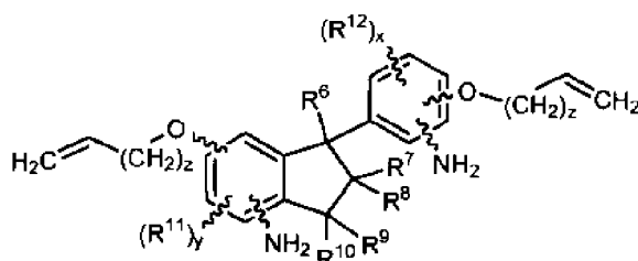
Struktur (I)
