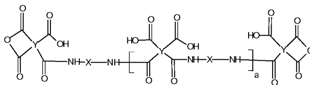
Structure (VIIb)
