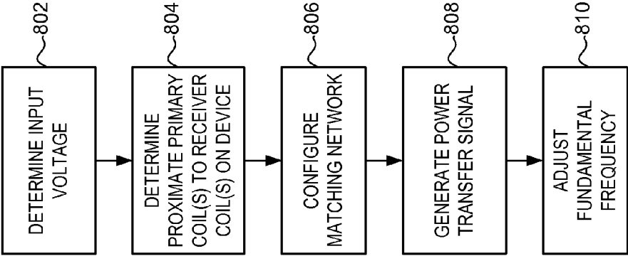
800 FIG. 8
