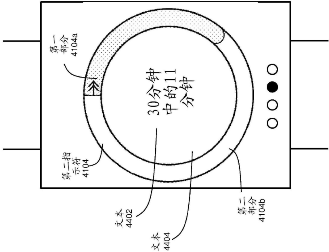
界面 4400
