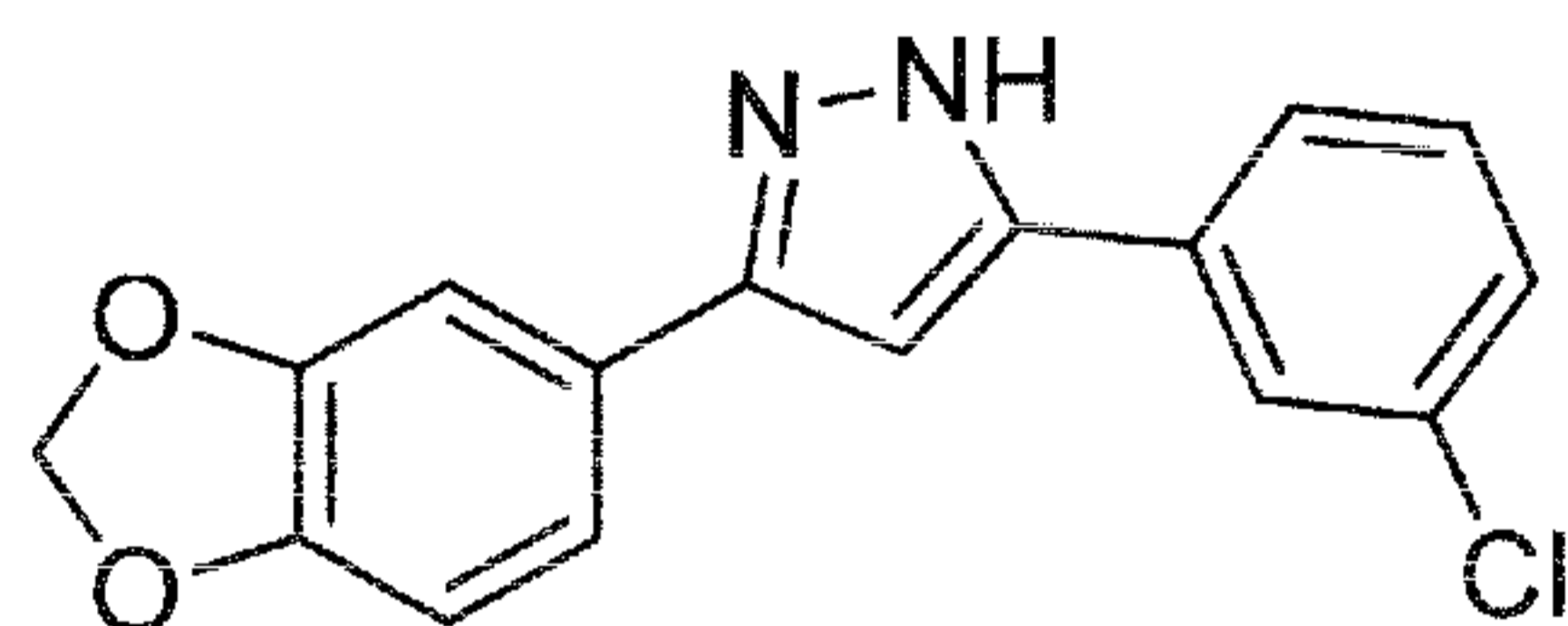
5-(3-Chlorophenyl)-3-(3,4-methylenedioxyphenyl)-1H-pyrazole
