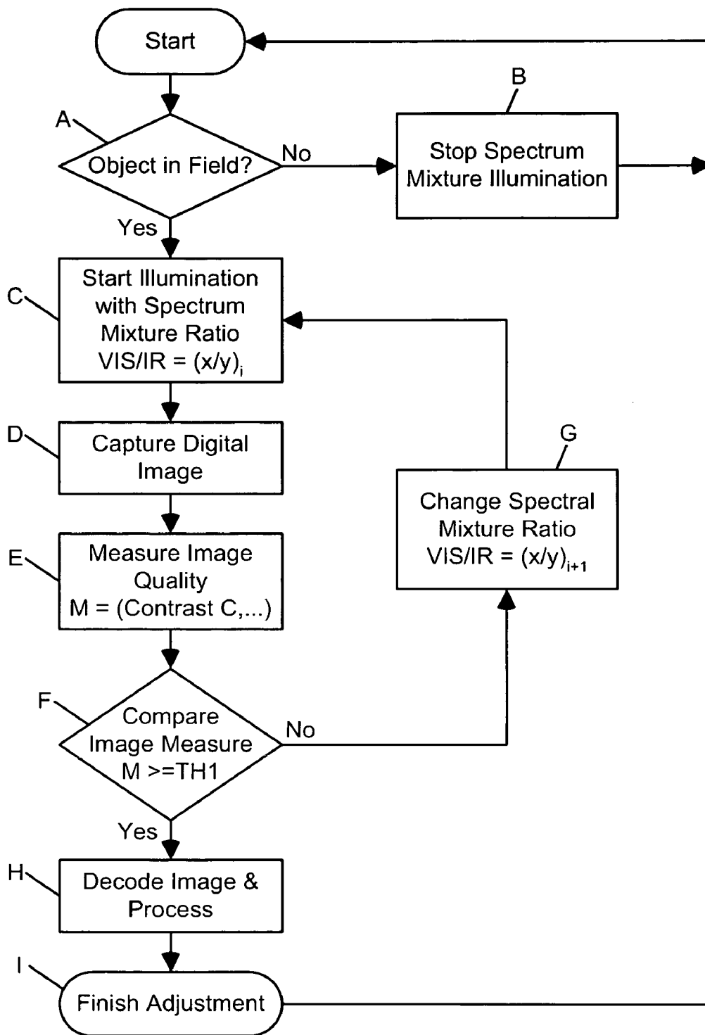
FIG. 5G2
