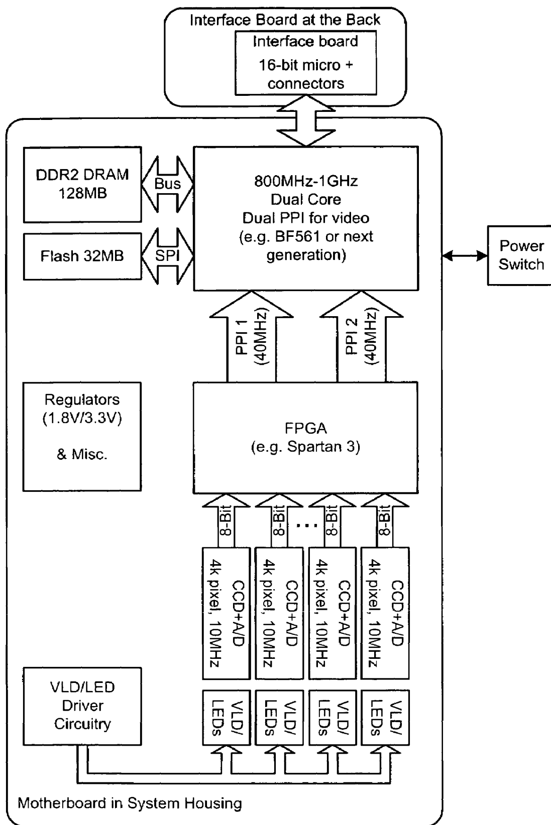
FIG. 7H
