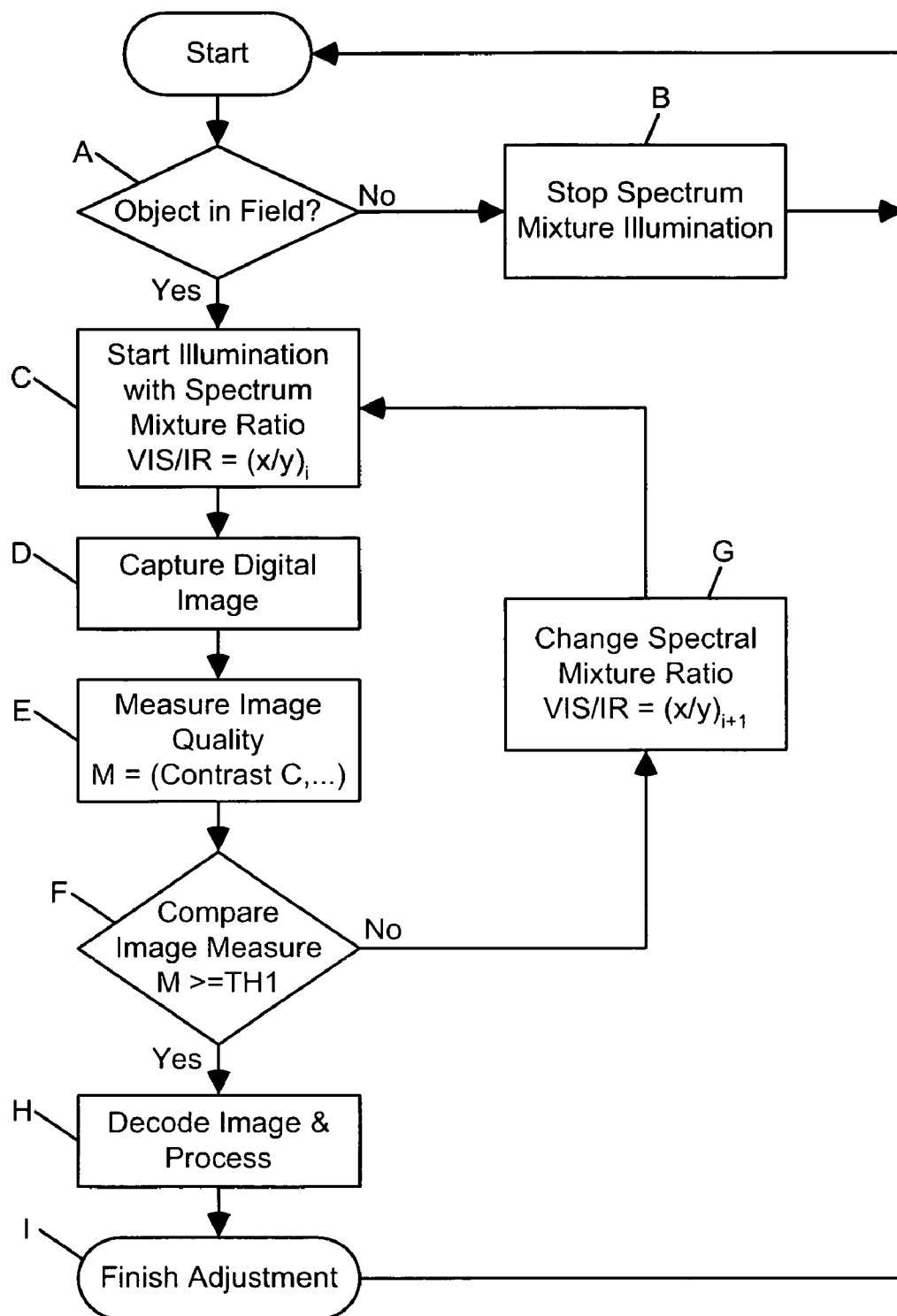
FIG. 5F2
