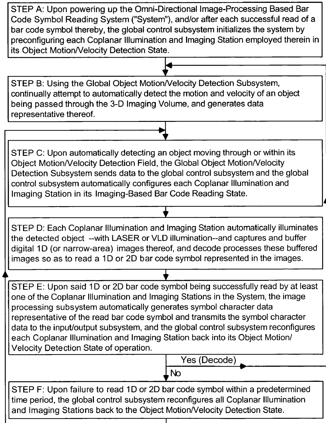
FIG. 7G
