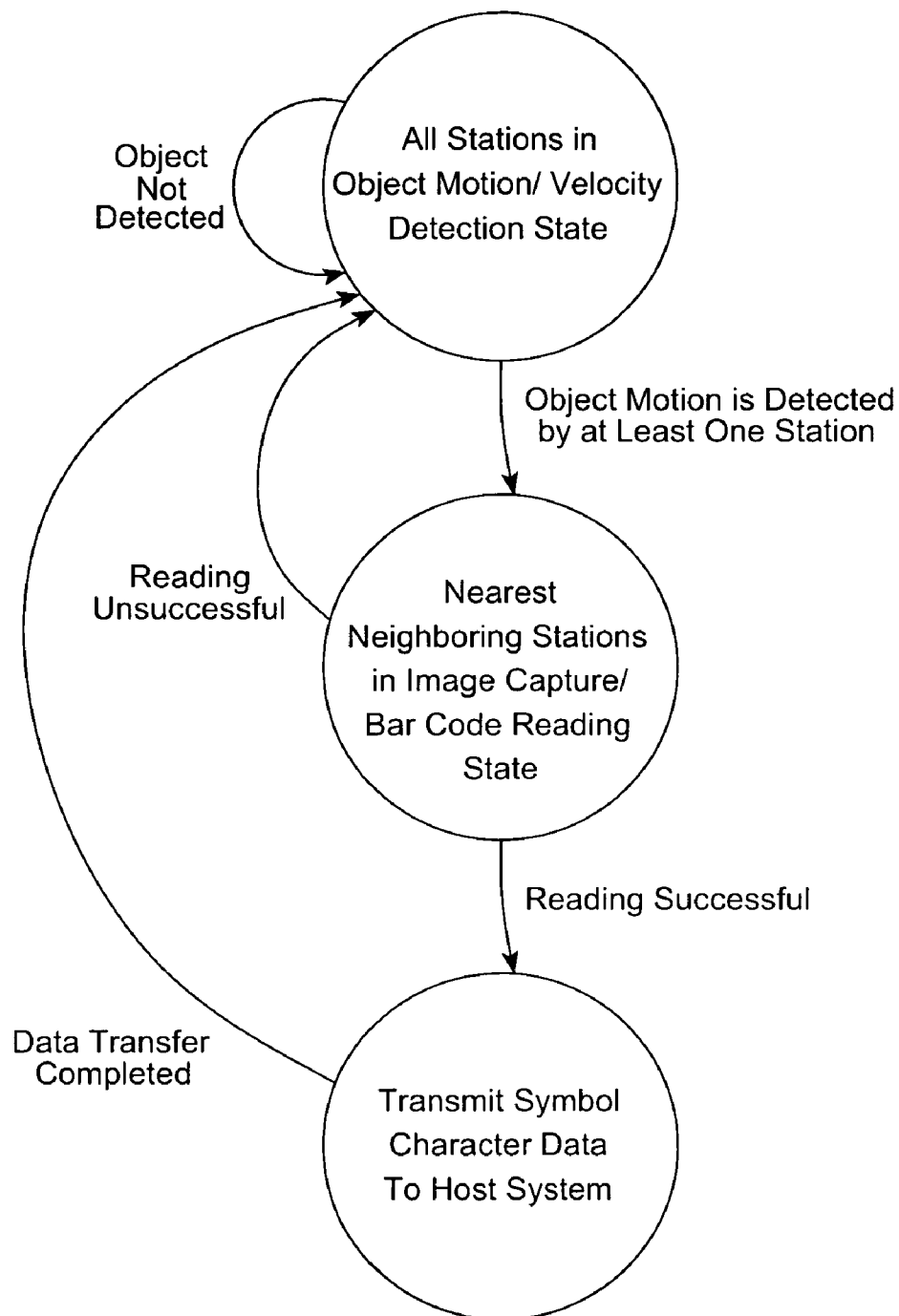
FIG. 8F2
