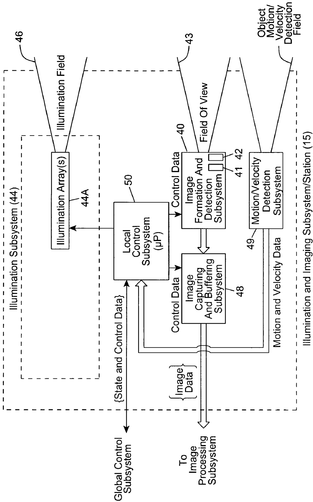
FIG. 5B
