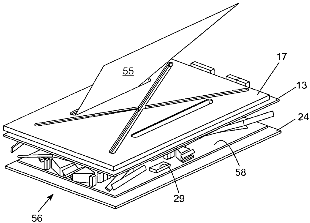
FIG. 3F
