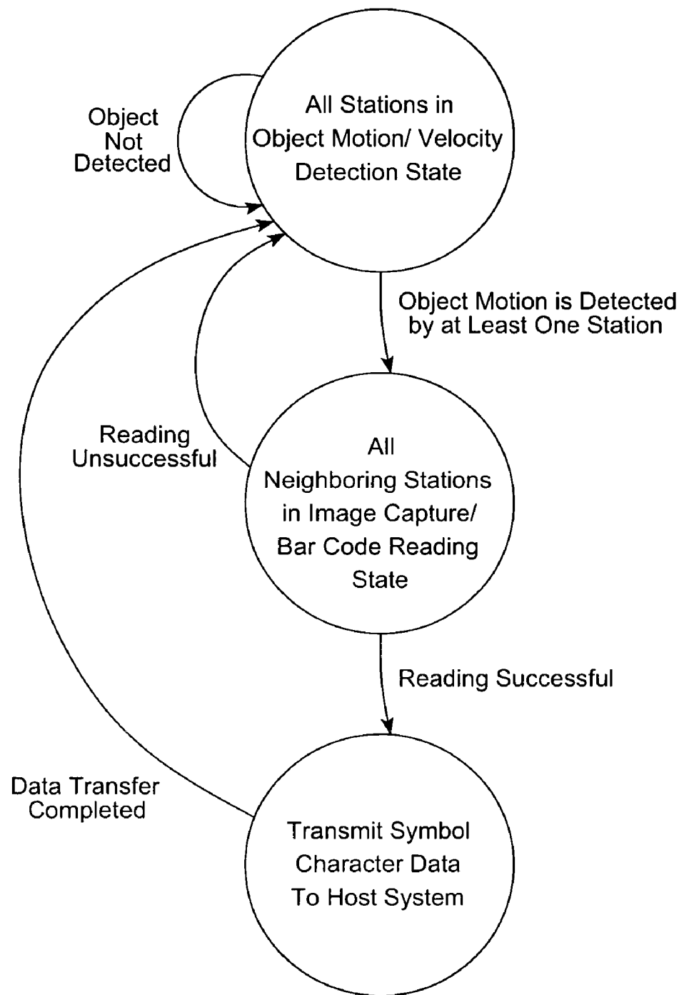
FIG. 8F3
