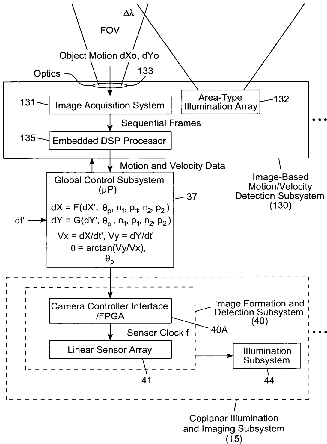
FIG. 7A3
