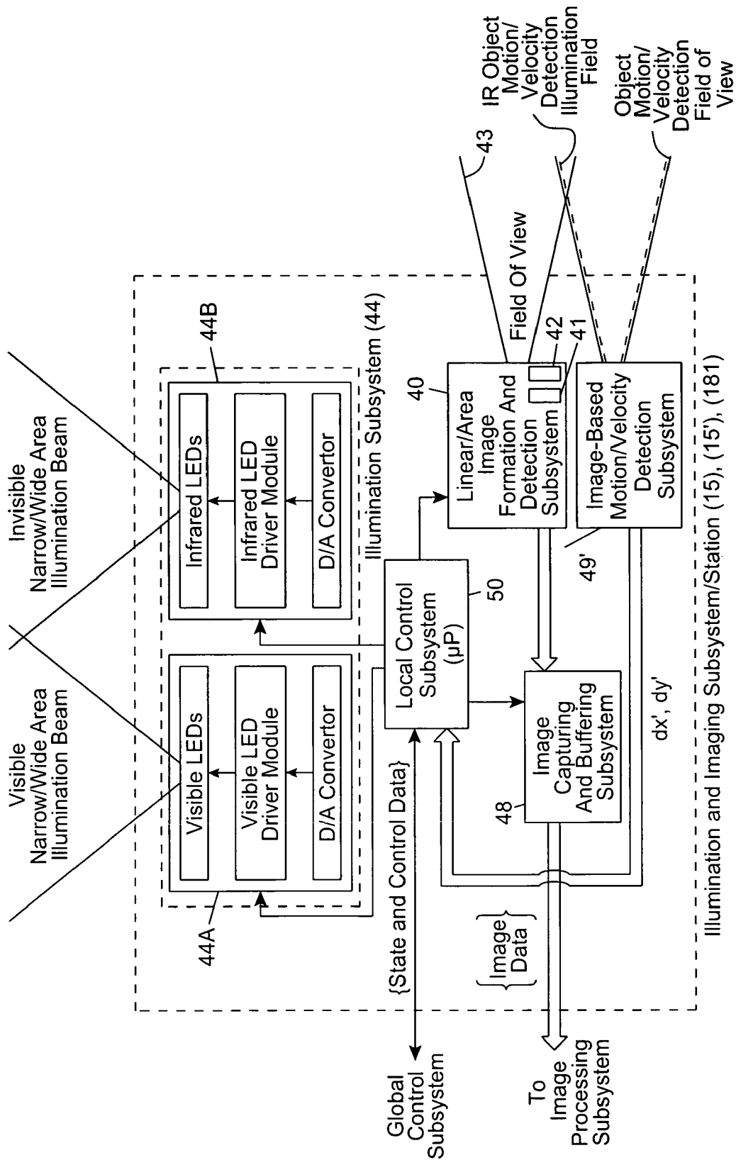
FIG. 5G1
