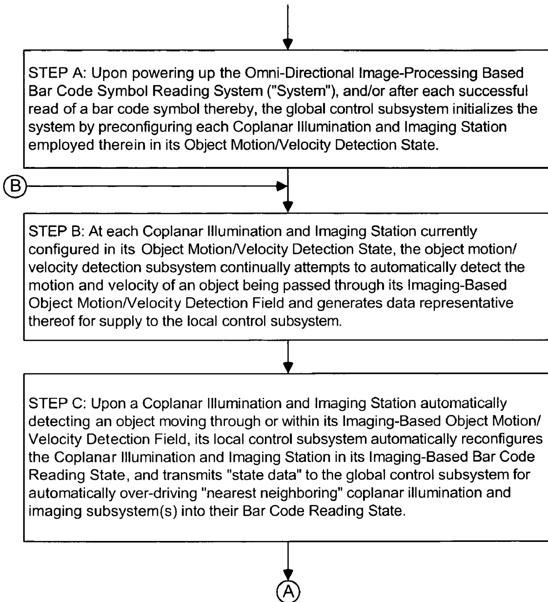
FIG. 6G2A
