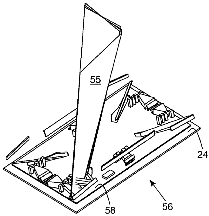
FIG. 4E
