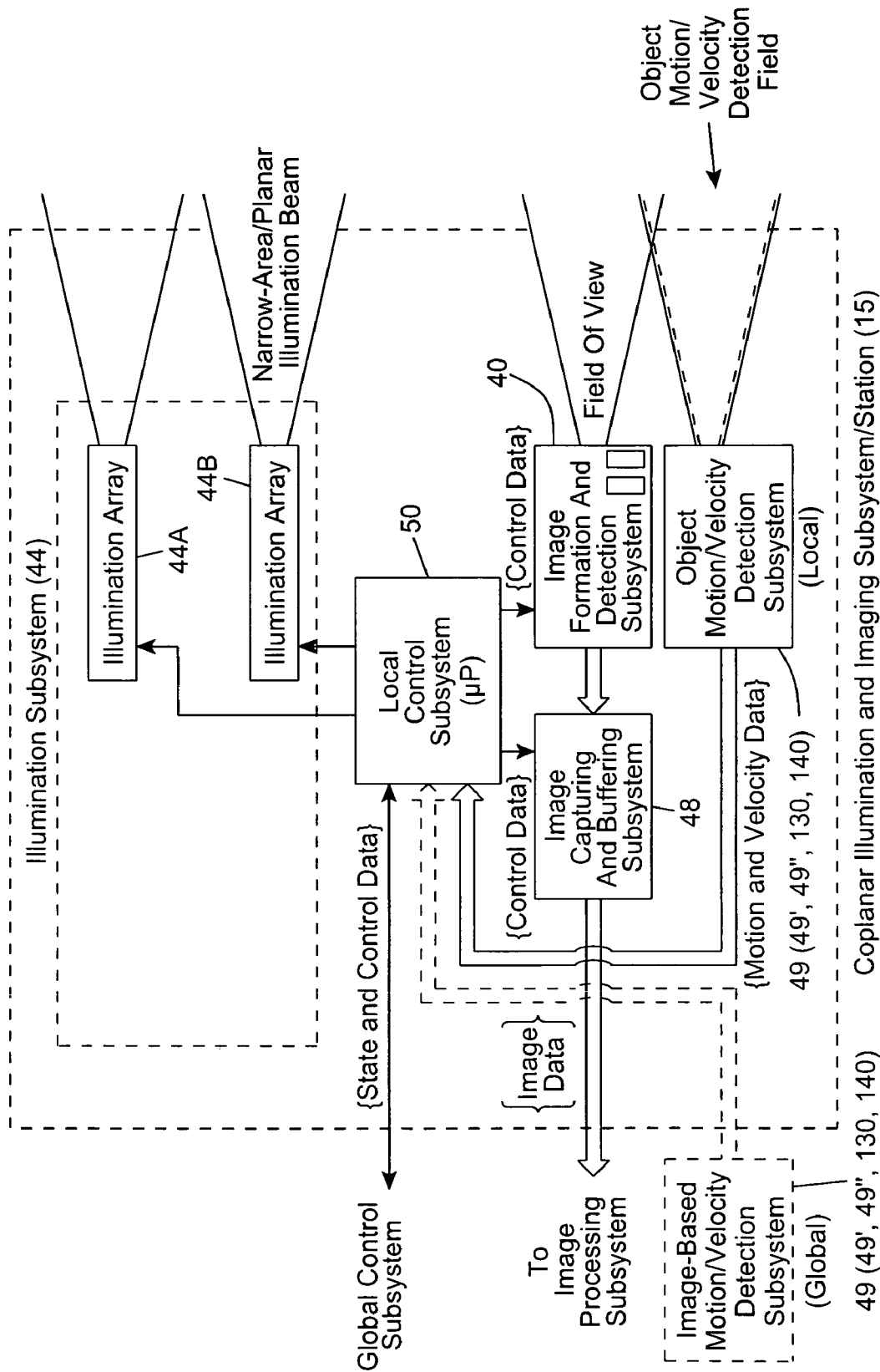
FIG. 9D
