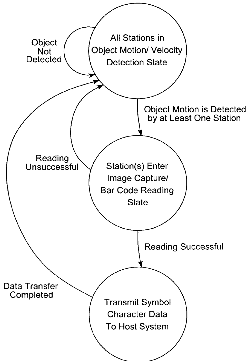
FIG. 8F1
