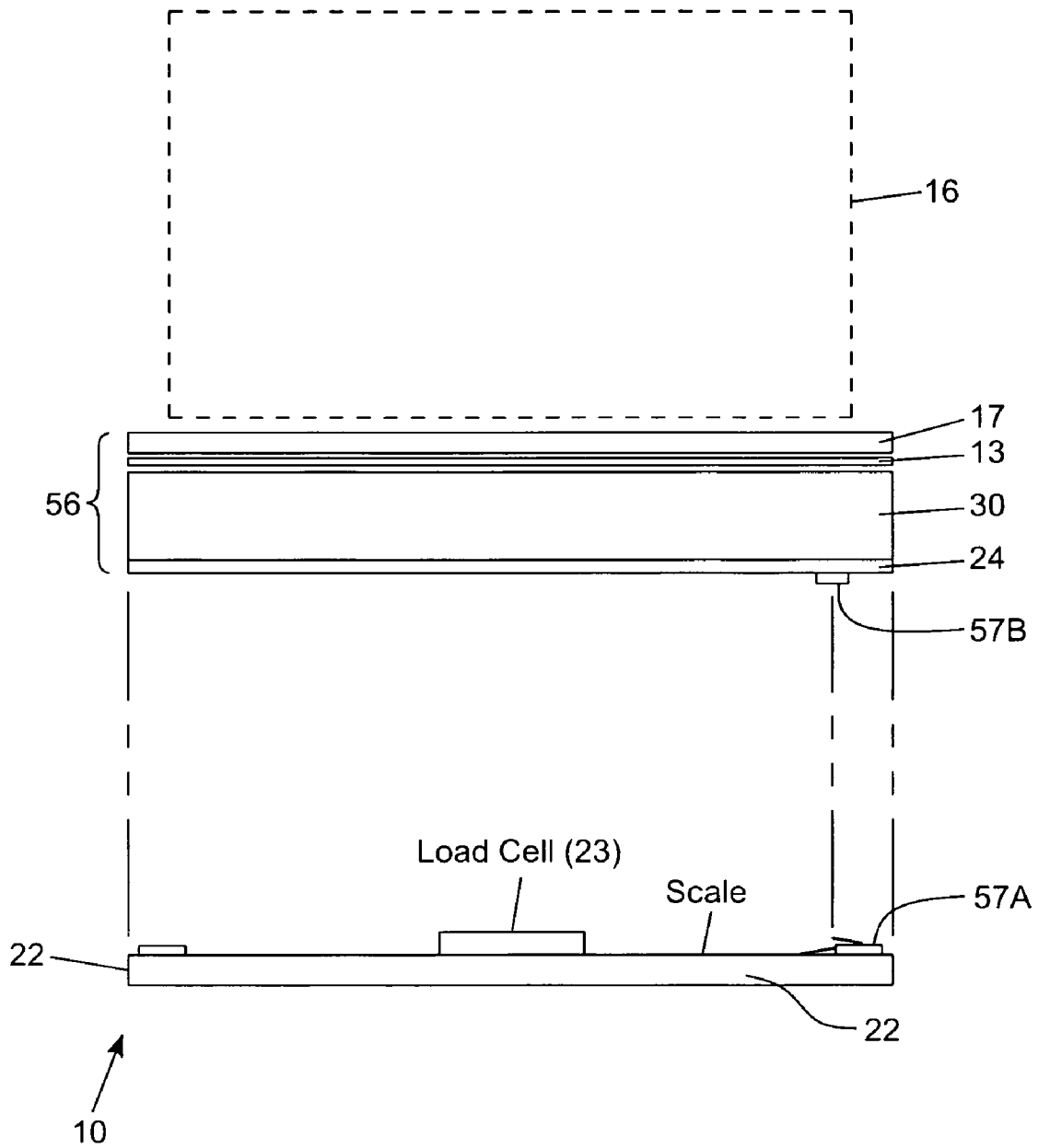
FIG. 2C
