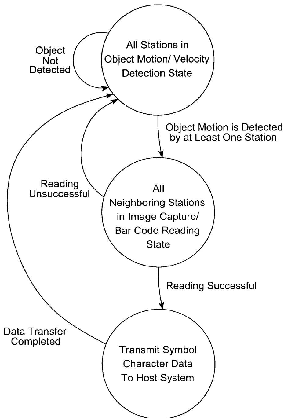
FIG. 9F3
