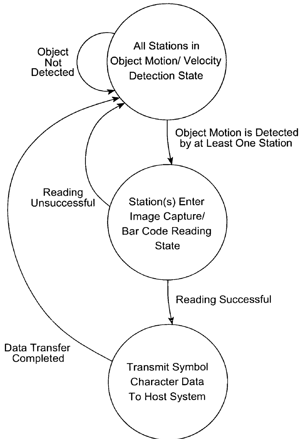
FIG. 9F1
