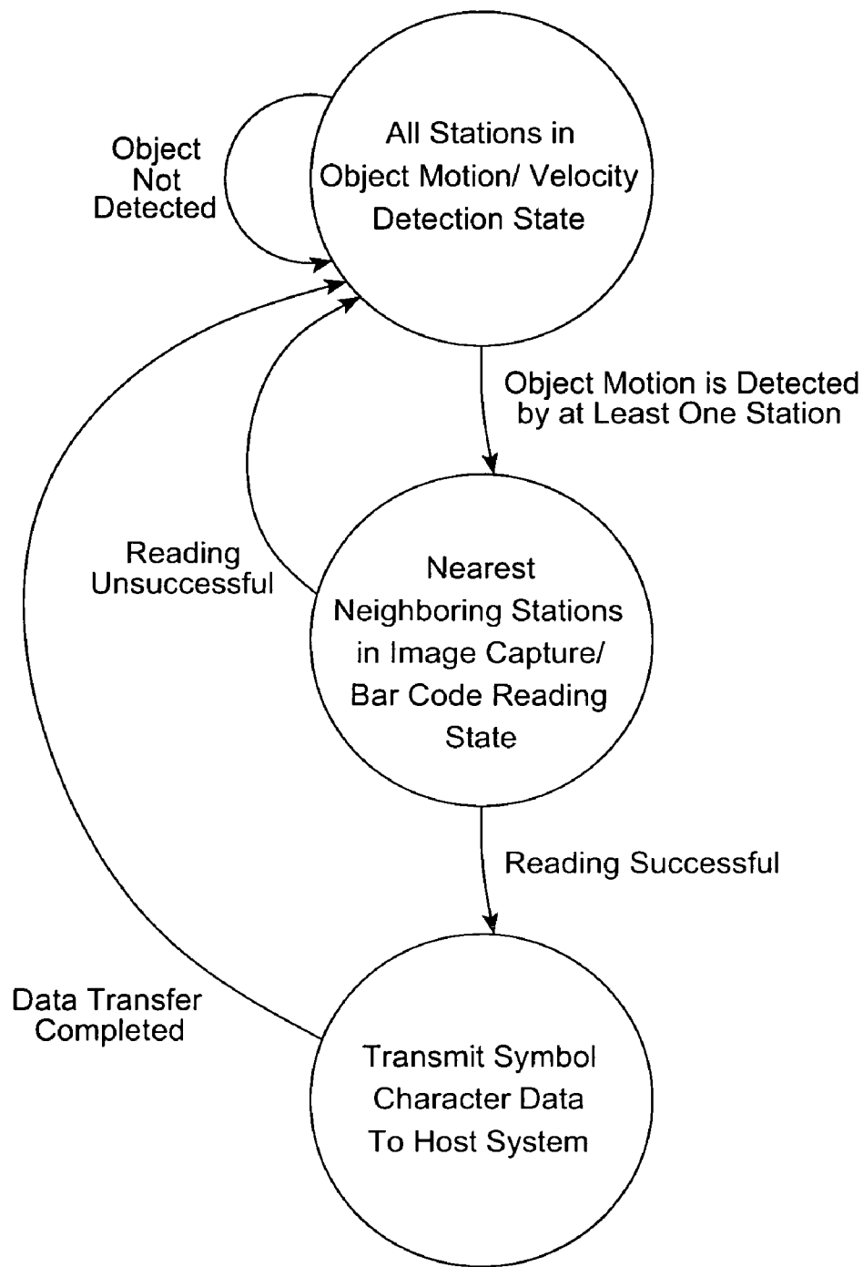
FIG. 9F2
