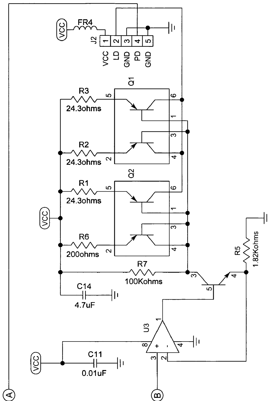
FIG. 5M2
