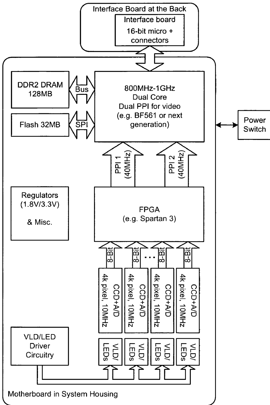
FIG. 6H
