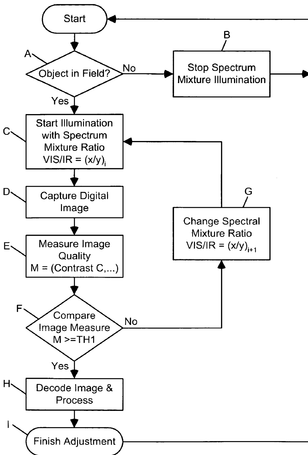
FIG. 5E2
