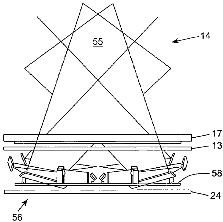
FIG. 3H
