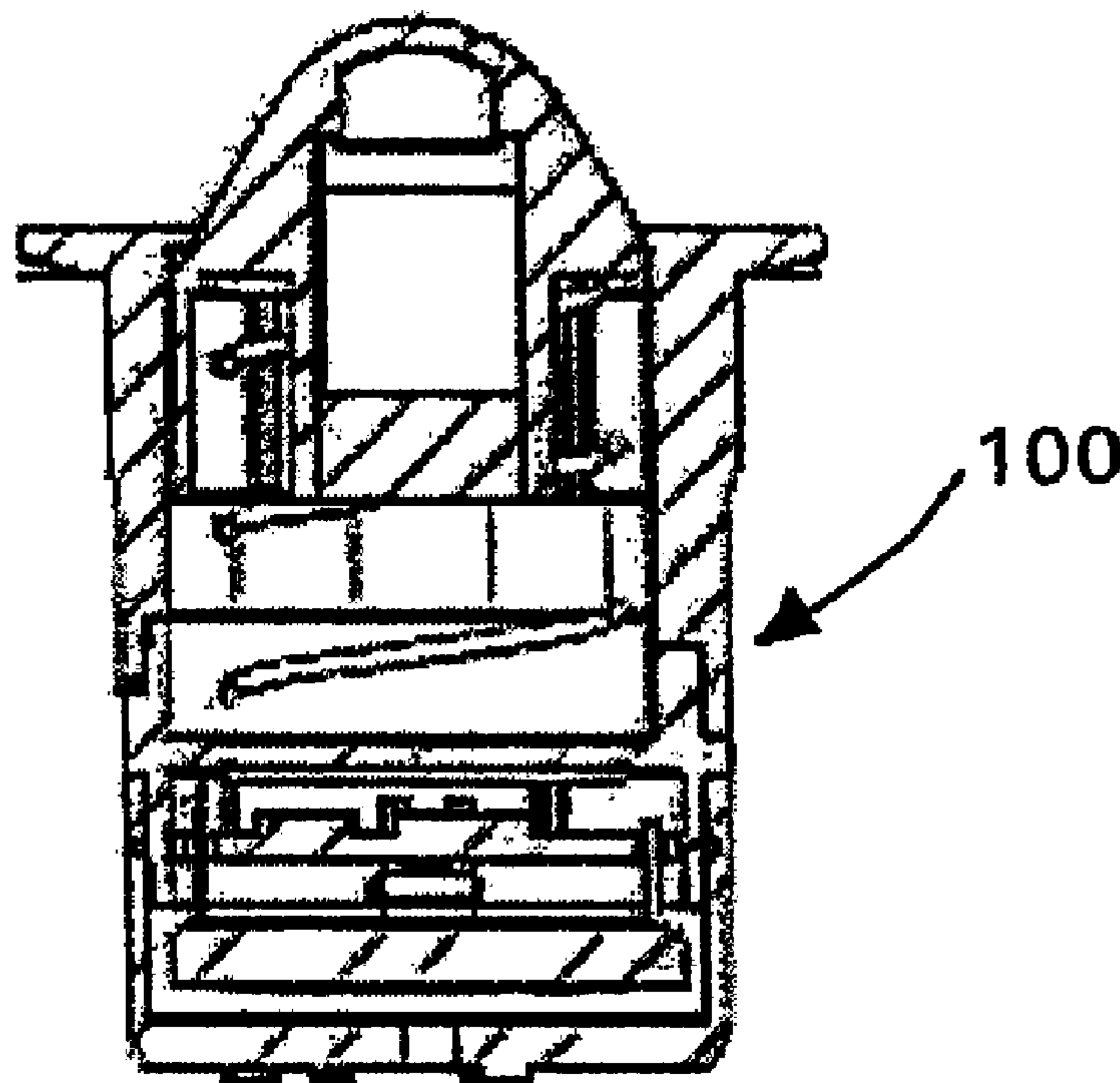
SECTION A-A
