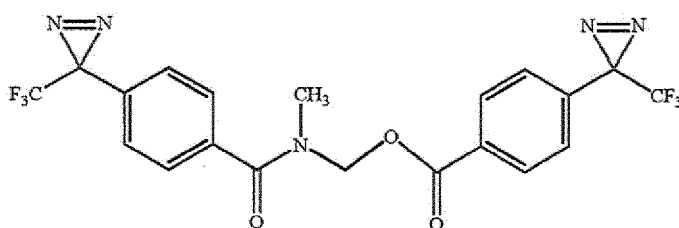
(N-méthyl-4-(3-(trifluorométhyl)-3H-diazirin-3-yl)benzamido)méthyle yl)benzoate ; et
