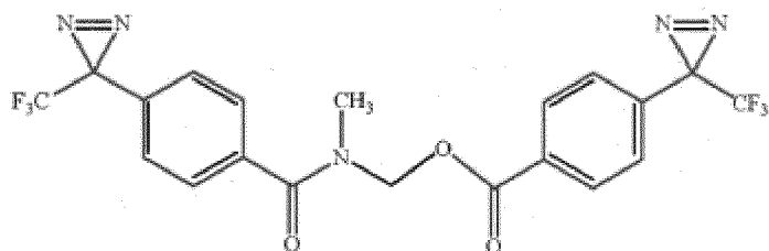
(N-Methyl-4-(3-(trifluormethyl)-3H-diazirin-3-yl)benzamido)methyl 4-(3-(trifluormethyl)-3H-diazirin-3-yl)benzoat; und
