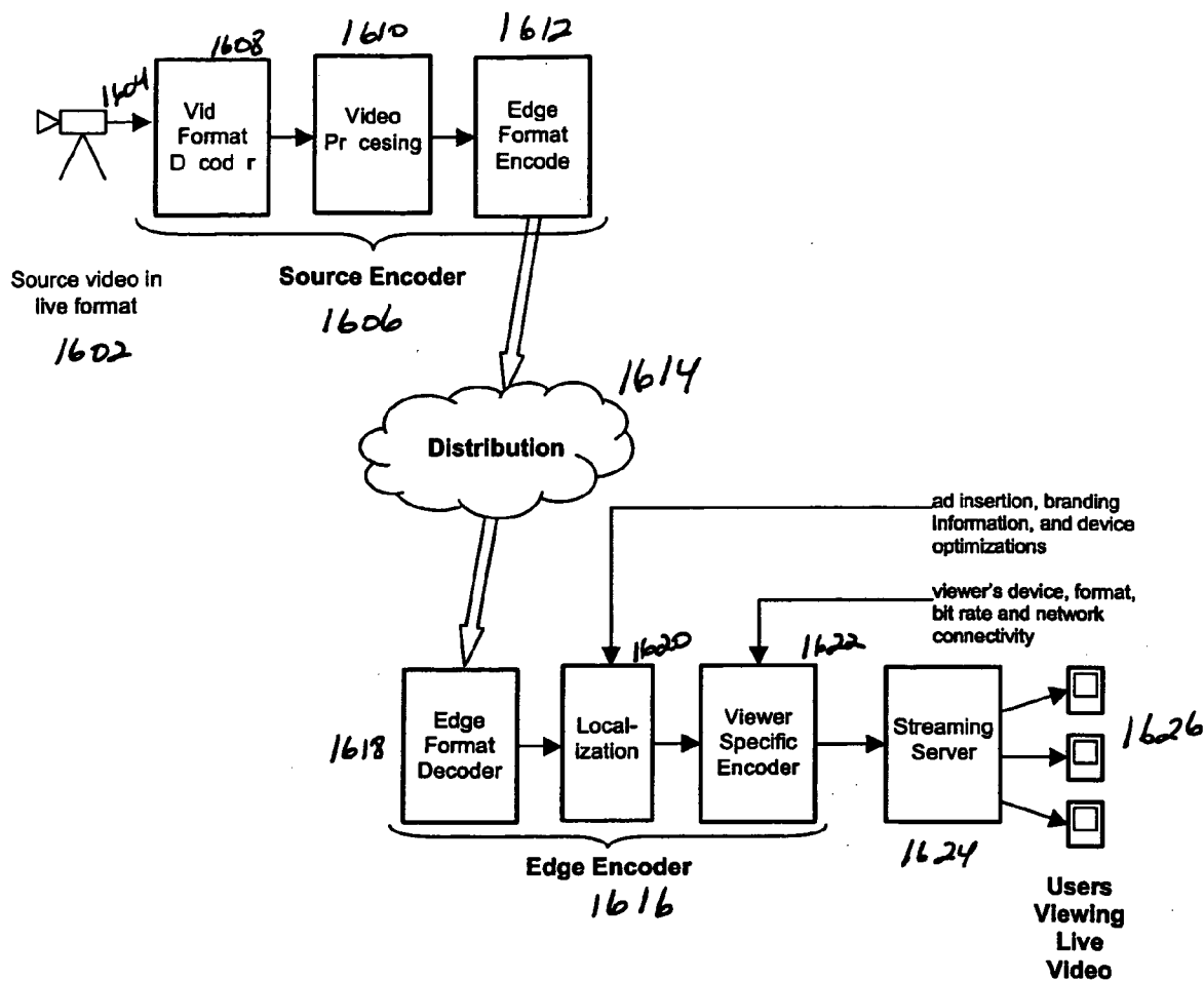
Figure 16: Edge Encoding
