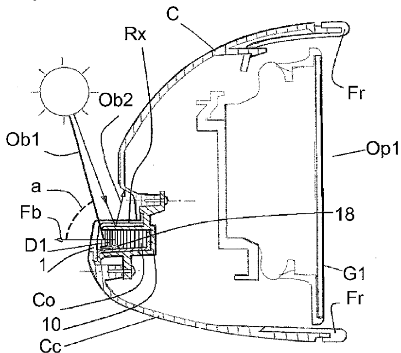
Fig.24, B-B
