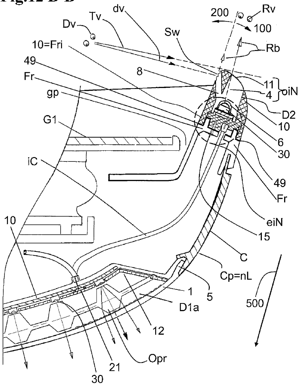
Fig.12 B-B
