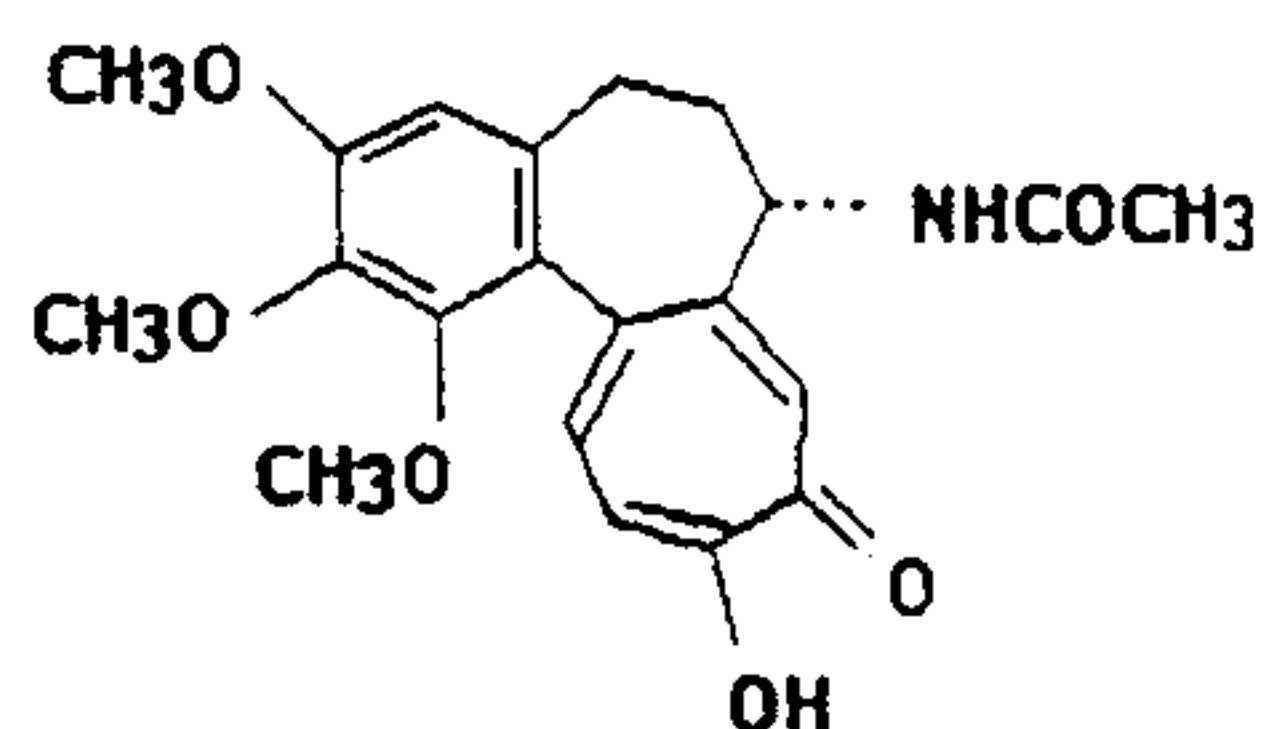
Colchicine
