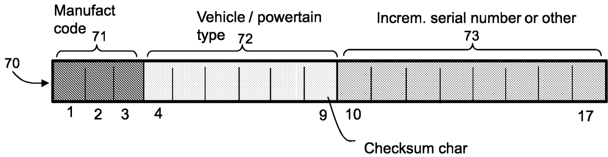
FIG. 3 VIN breakdown
