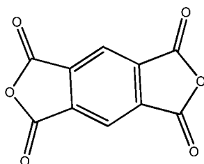
Formule III(a)
