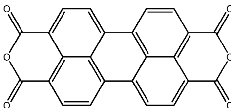
Formule III(b)
