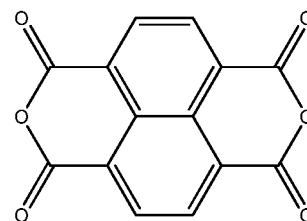
Formule III(c)
