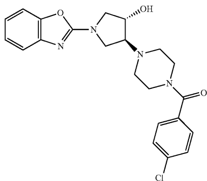
1-(1,3-benzoxazol-2-yl)-4-[4-(4-chlorobenzoyl)piperazin-1-yl]pyrrolidin-3-ol
