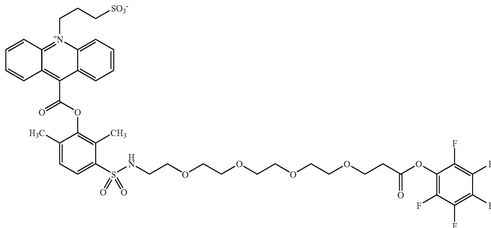
SPAЕ-PEO4-PFP
