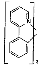
Ir(ppy) 3
