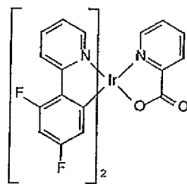
Ir(pic)
