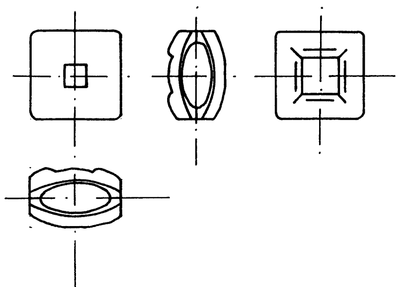
Rys.2. Rzuty spinki
